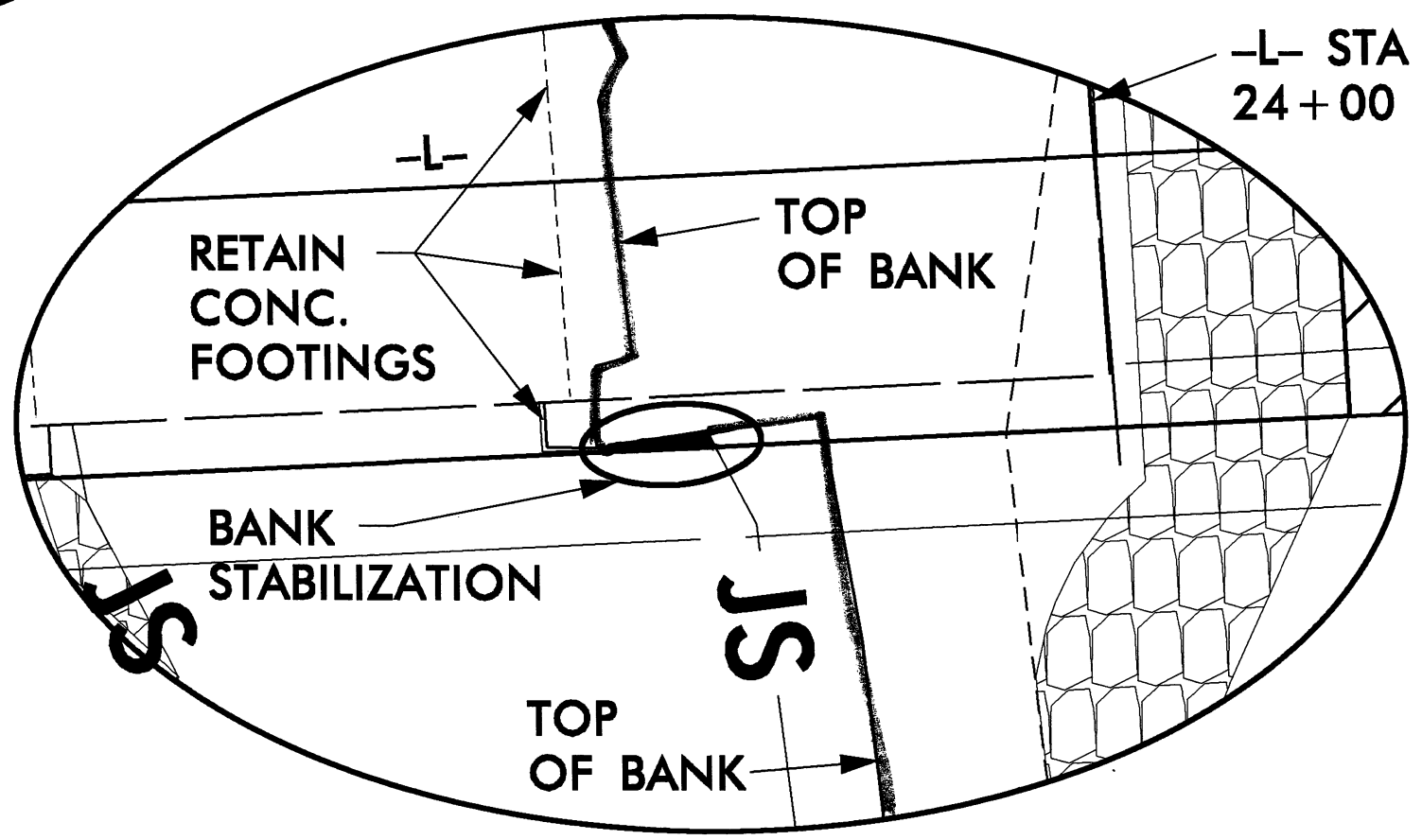
DETAIL 2 -L- STA 23+75 RT
