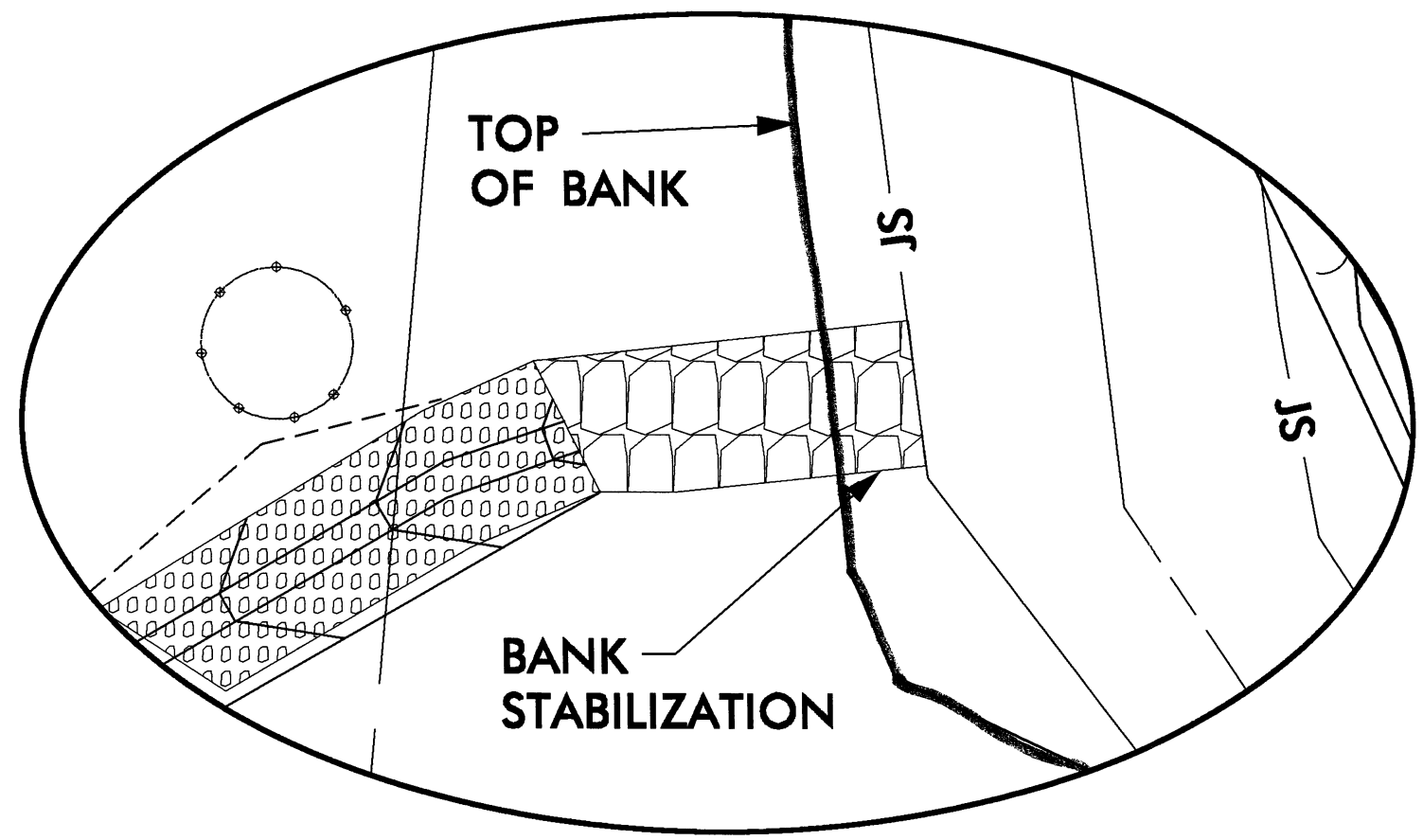
DETAIL 1 -L- STA 23+23 LT
