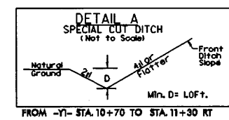
FROM -YI- STA. 10+70 TO STA. 11+30 RT
