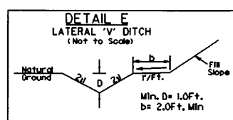
FROM -L- STA. 13+75 TO STA. 14+40 LT
