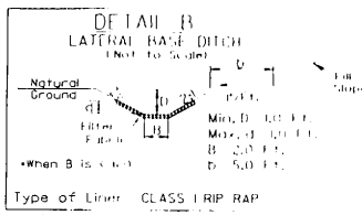
FROM STA. 16+00 TO STA. 16+50 LT. -L-
