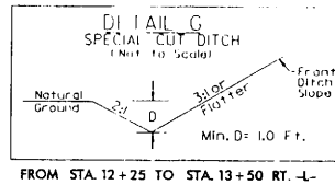
FROM STA. 12+25 TO STA. 13+50 RT. -L-
