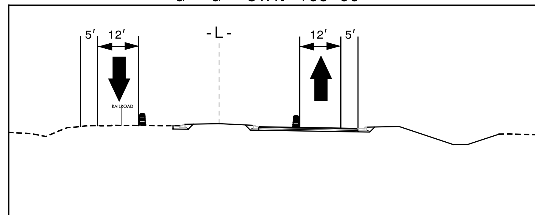
G''' - G''' STA. 105+00
