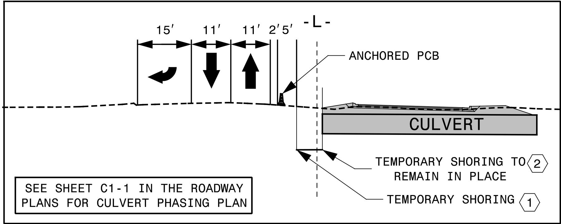
A-A STA. 26+50
