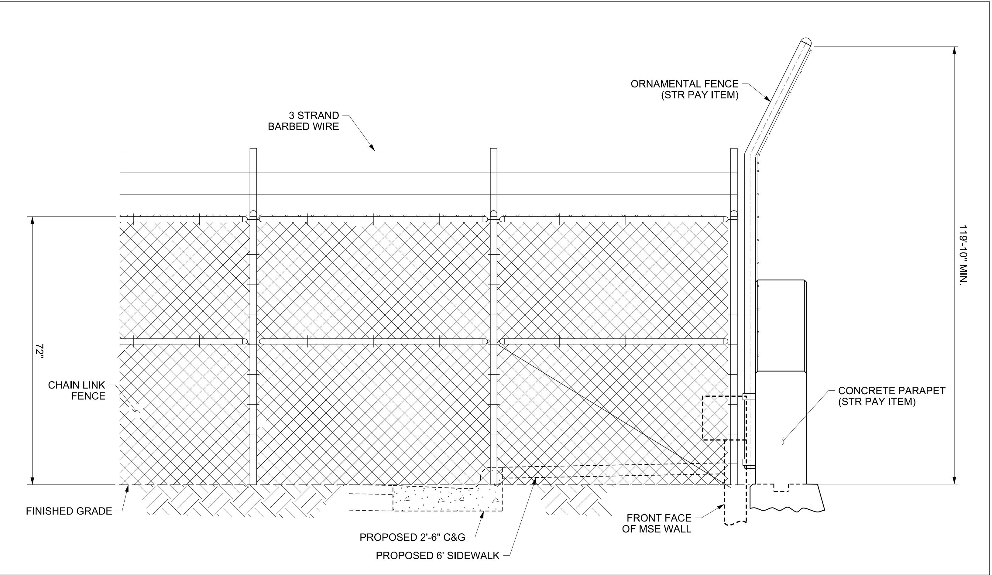
SECTION A-A
