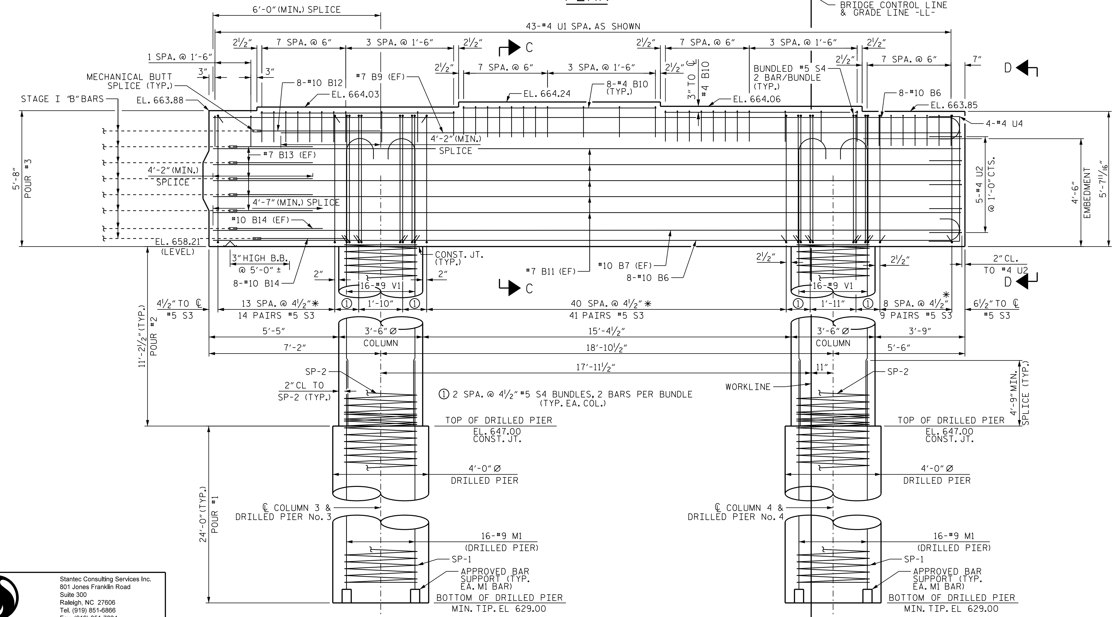
ELEVATION
