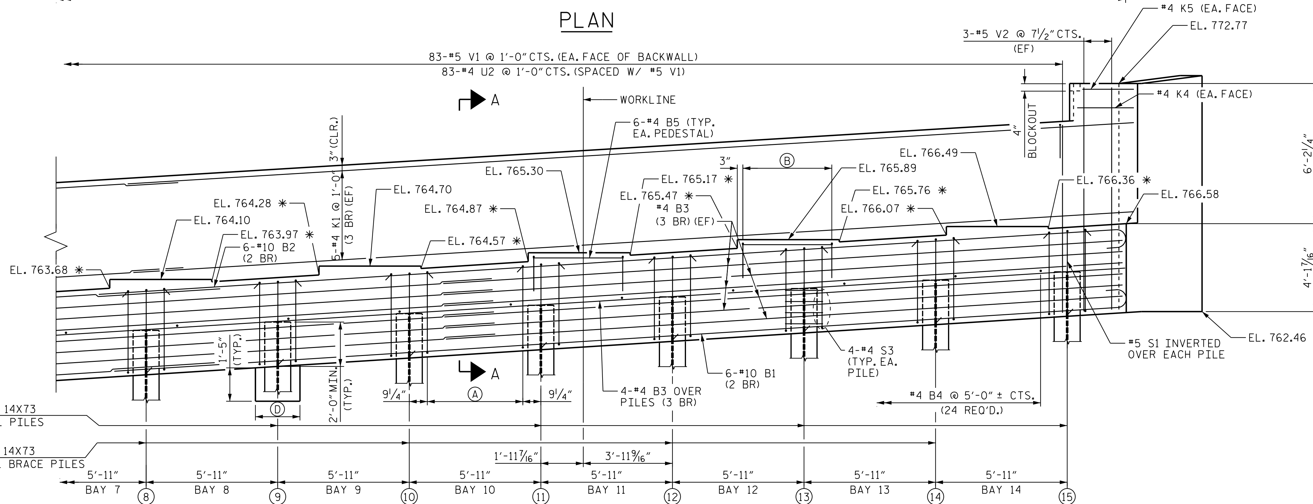
ELEVATION
