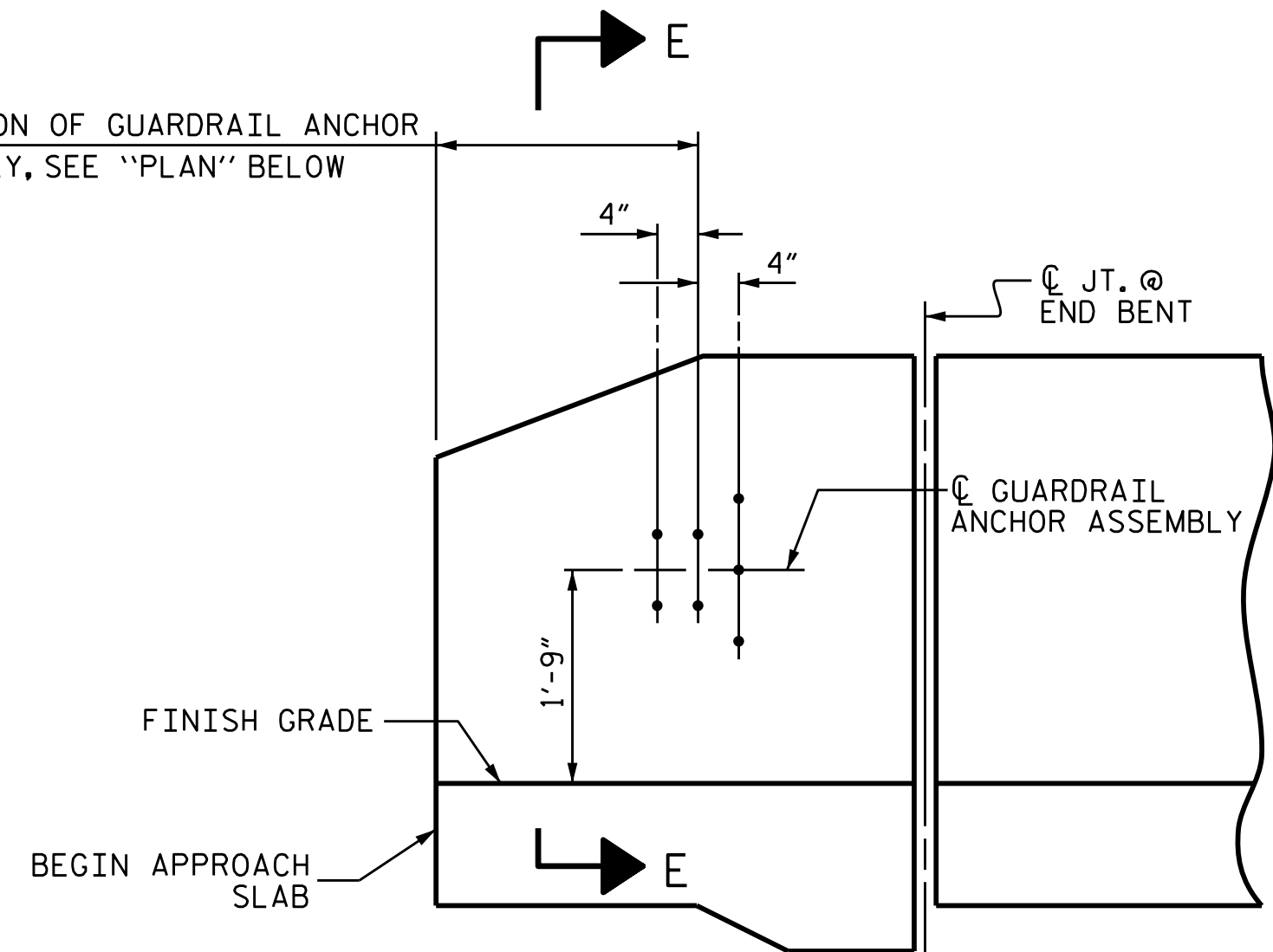
ELEVATION
