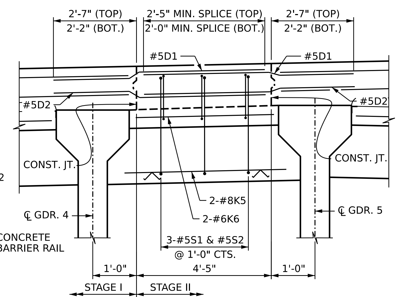
CLOSURE POUR DETAIL
