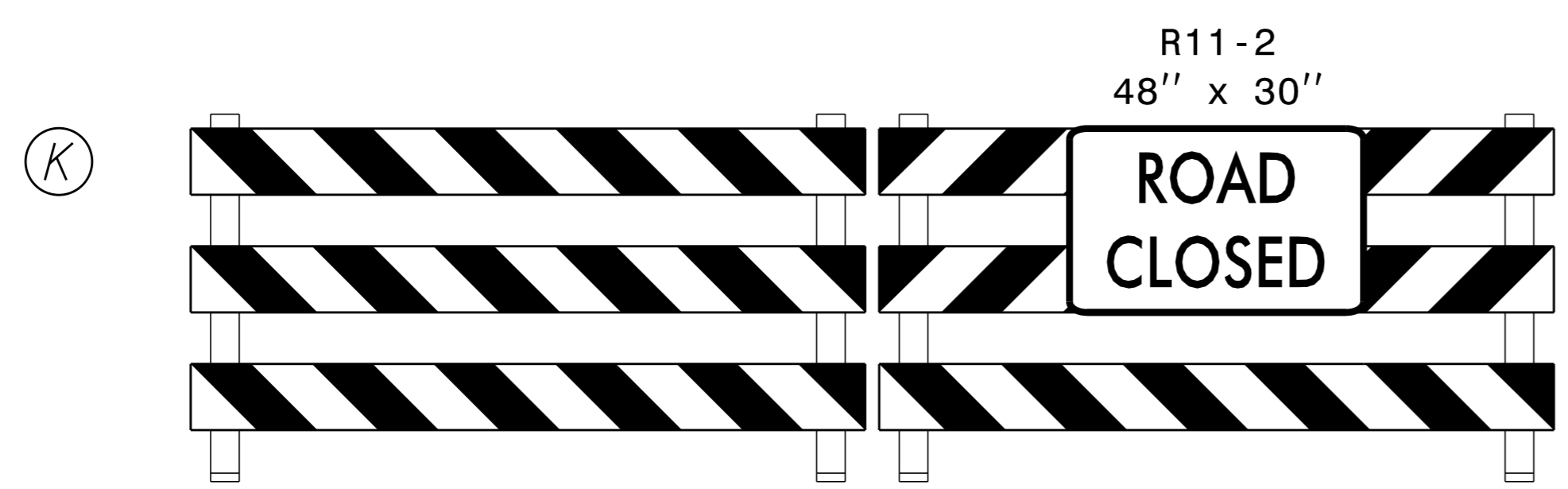
TYPE III BARRICADE(S)
