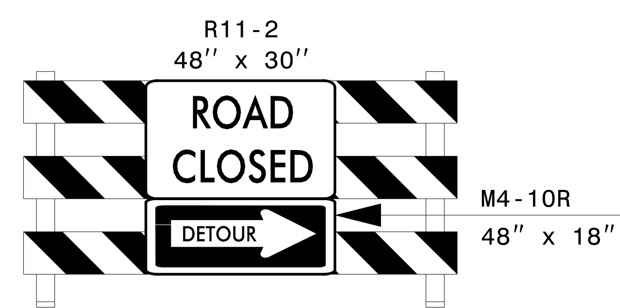
TYPE III BARRICADE
