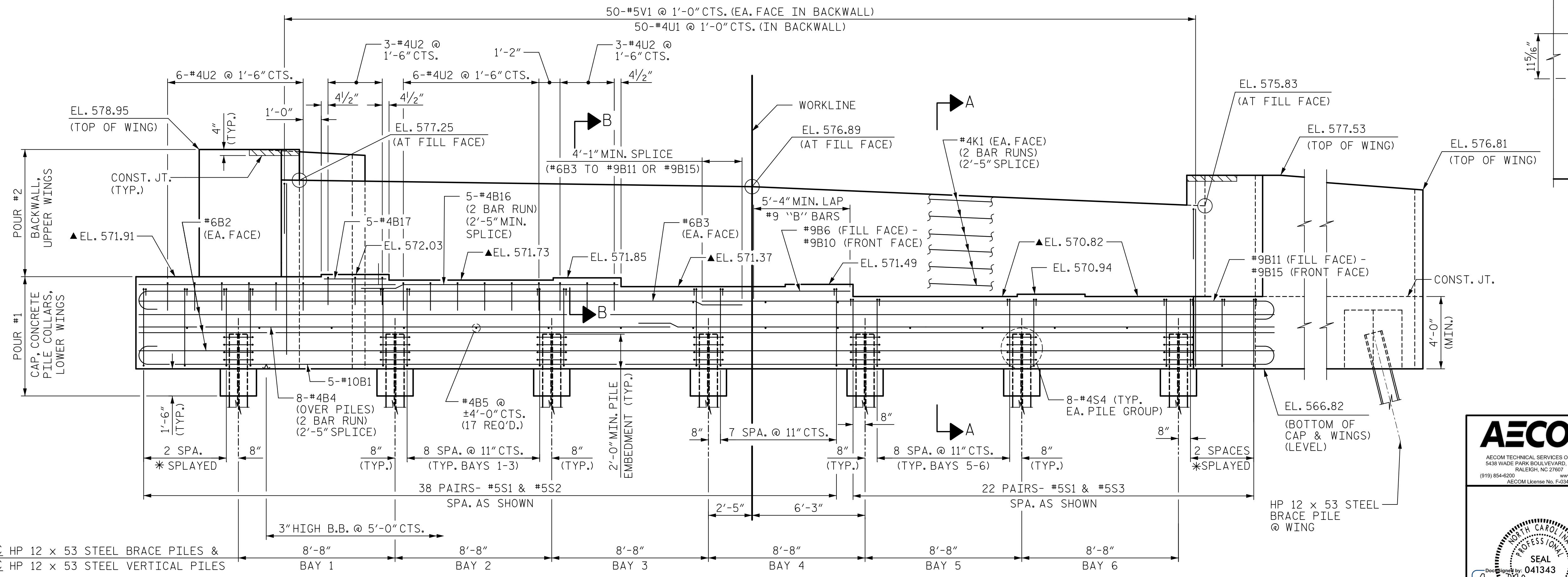
ELEVATION
