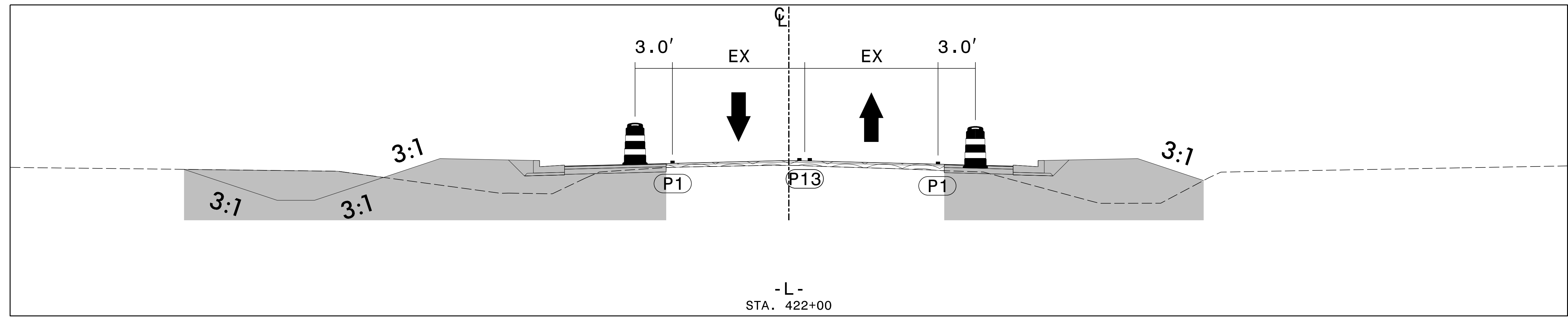
J1 36 76 STA. 422+00 -L- CUT SECTION
