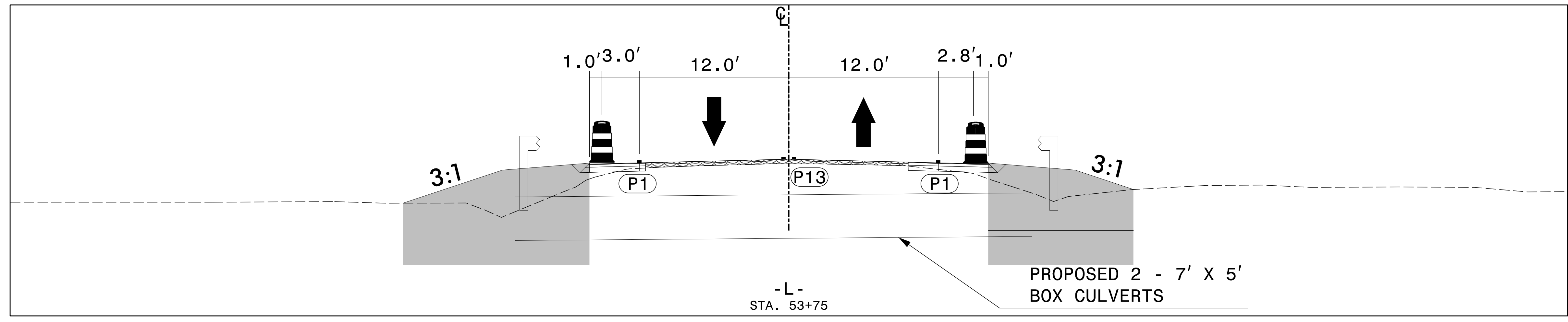
C1 08 | 69 STA. 53+75 -L- CUT SECTION
