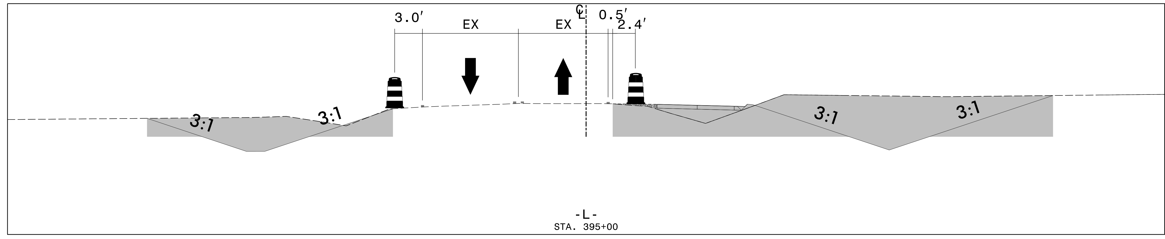
I 1 34 | 75 STA. 395+00 -L- CUT SECTION
