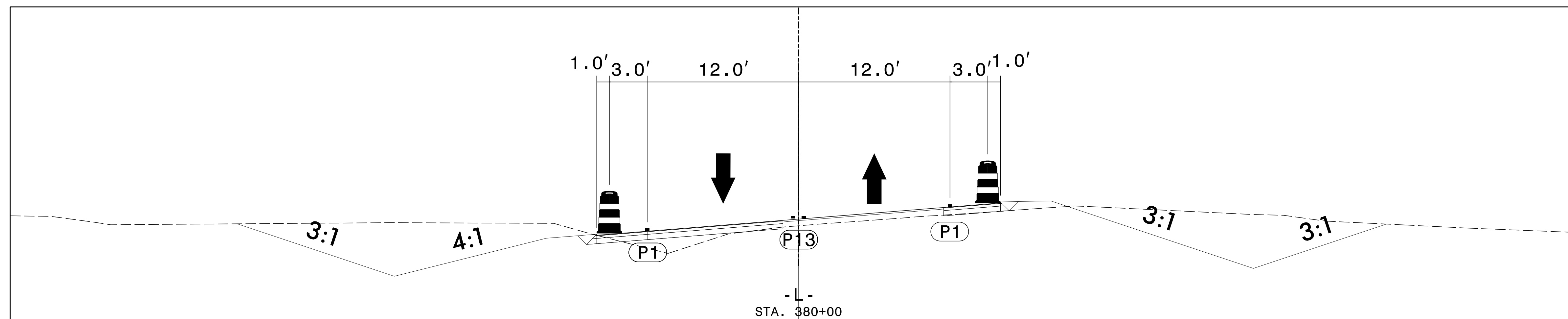
H2 STA. 380+00 -L- 63 | 74 CUT SECTION
