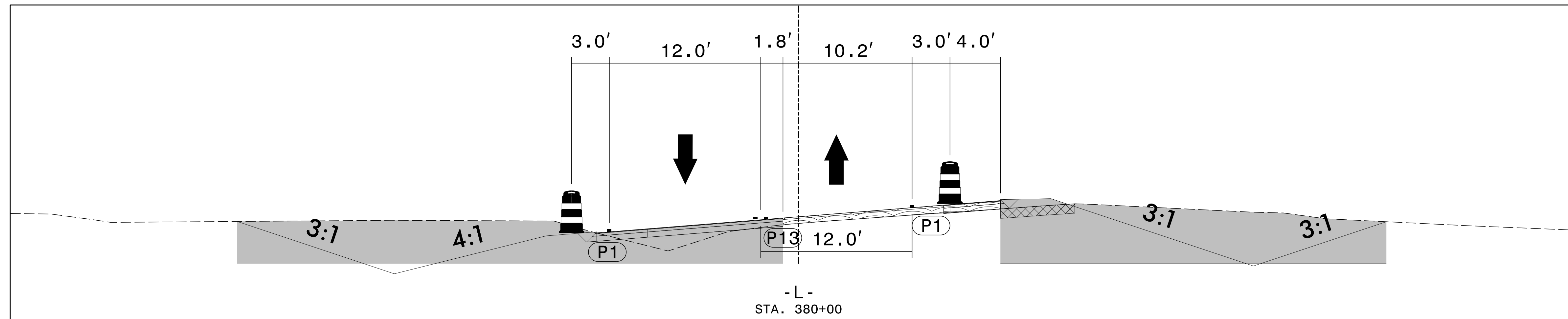
H1 STA. 380+00 -L- 33 | 74 CUT SECTION
