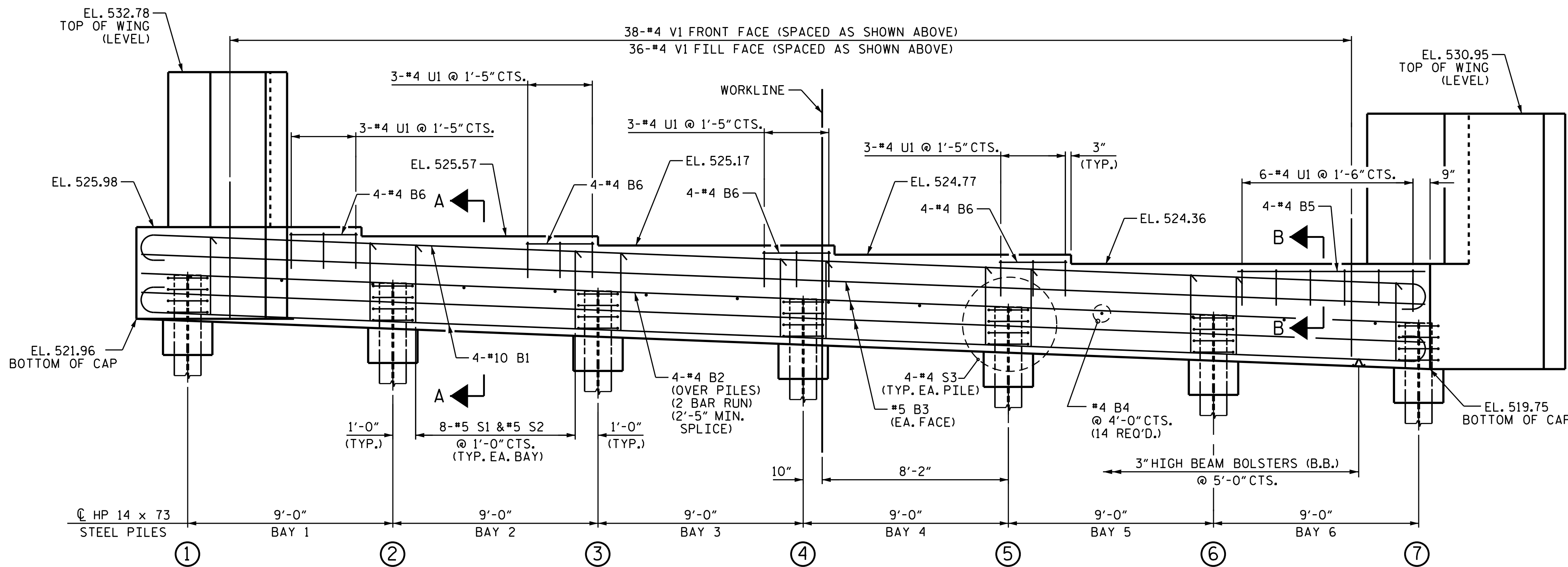
ELEVATION
