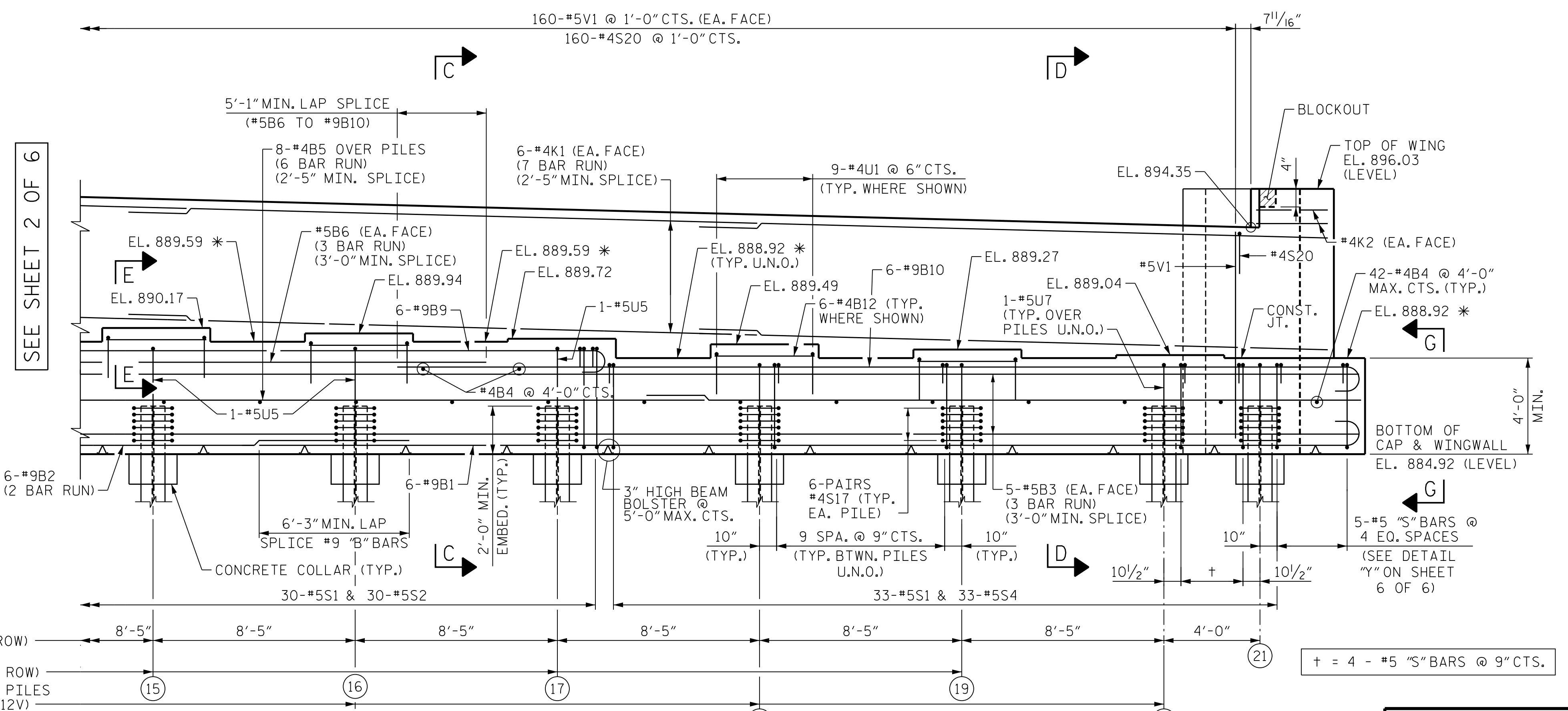
ELEVATION
