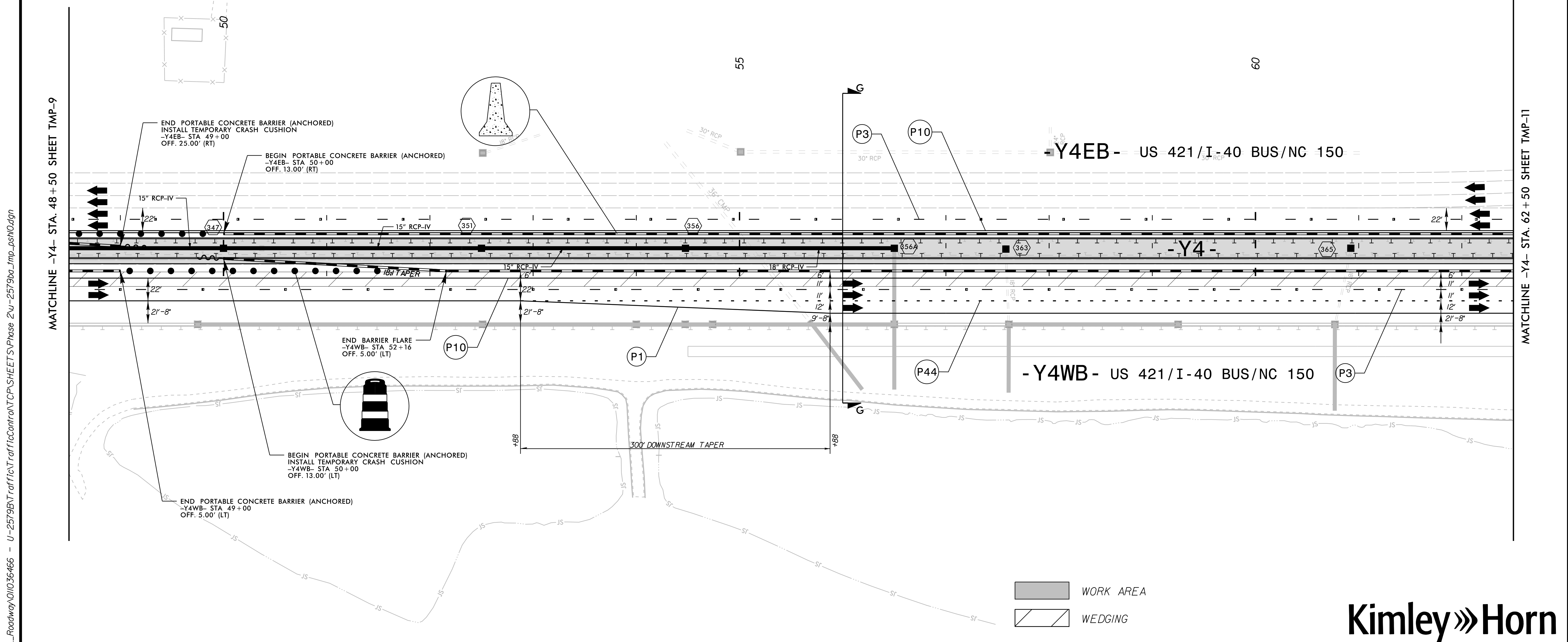
PHASE 2 SECTION G-G STA. 56+00
