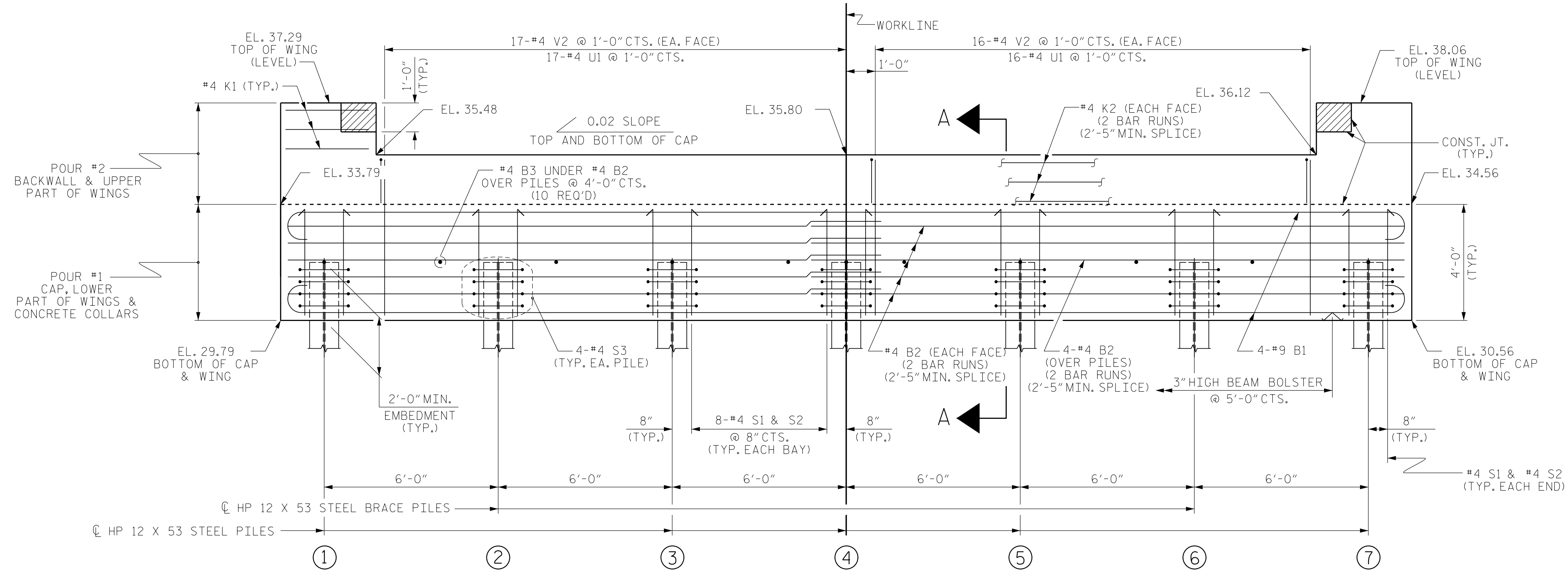
ELEVATION
