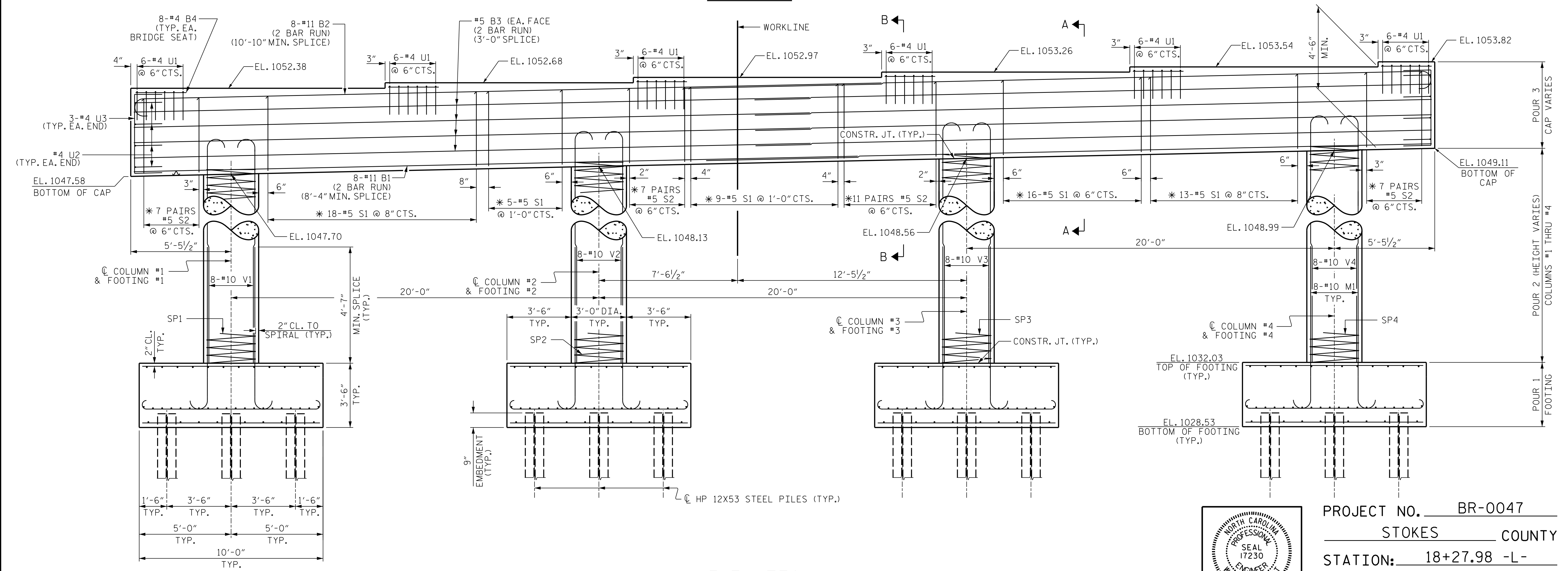
ELEVATION
