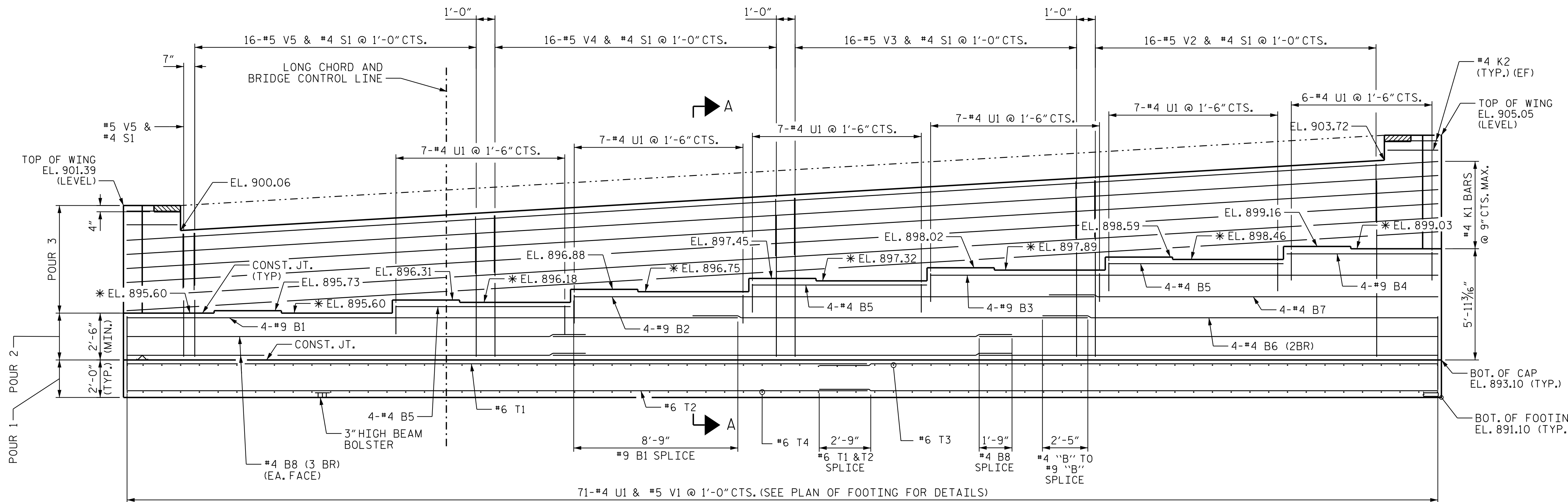
ELEVATION
