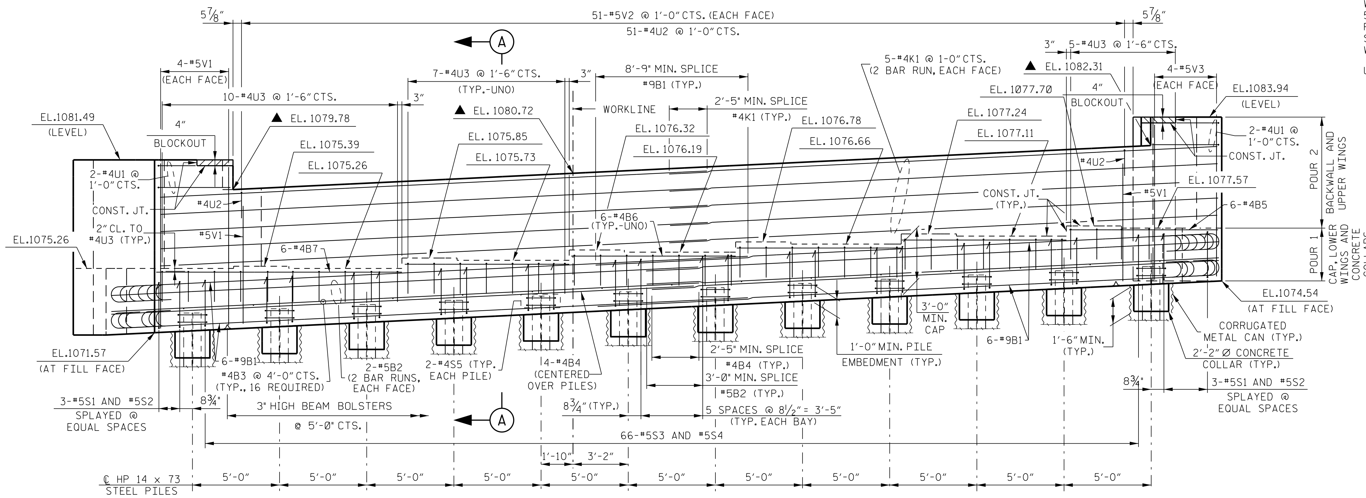
ELEVATION
