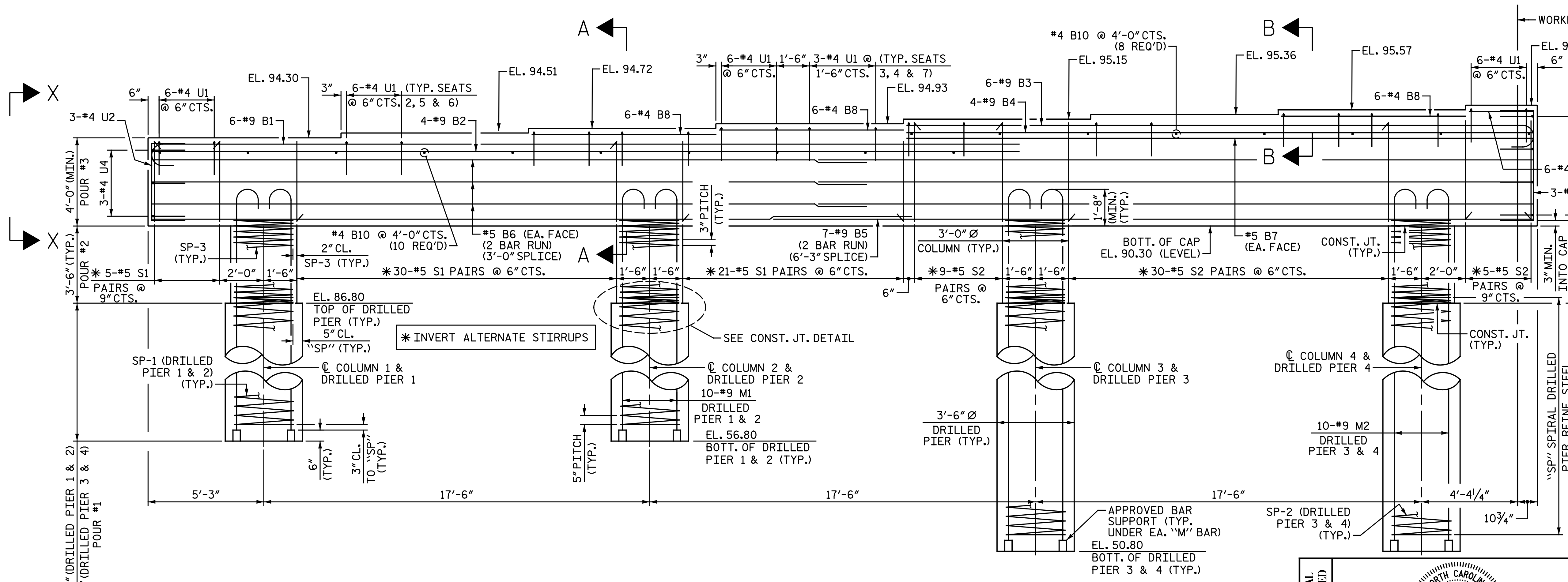
ELEVATION
