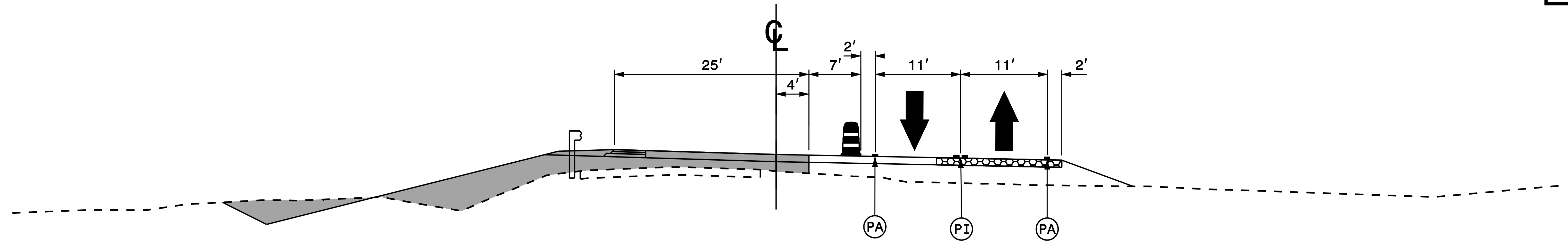
SECTION TMP-21A -Y7A- STA. 30+50 +/-
