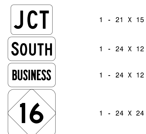
ONE "U" POST PER SIGN
