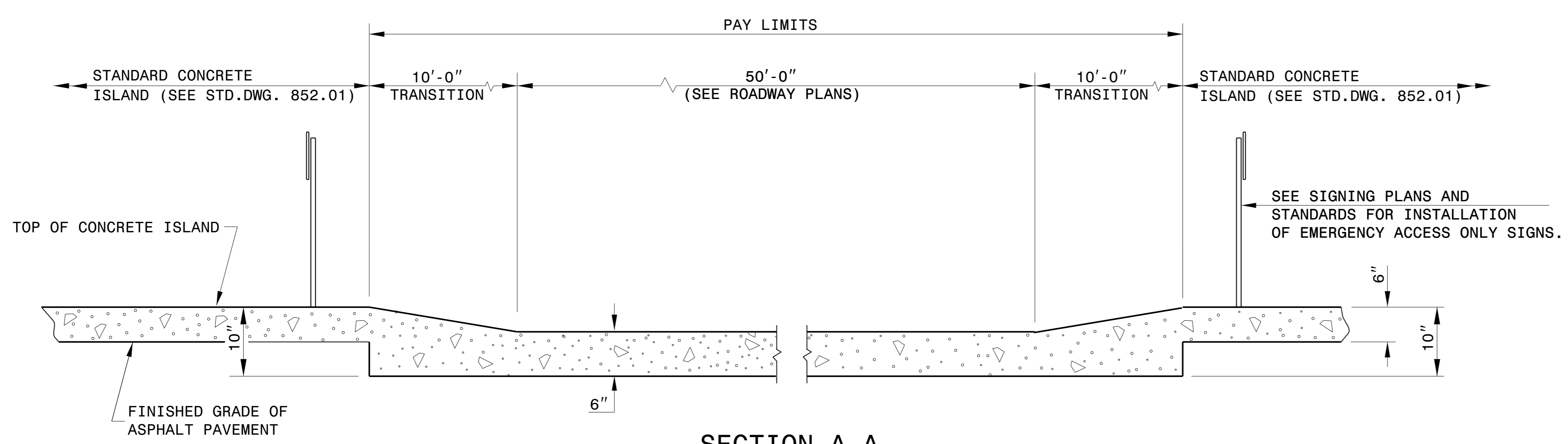
SECTION A-A
