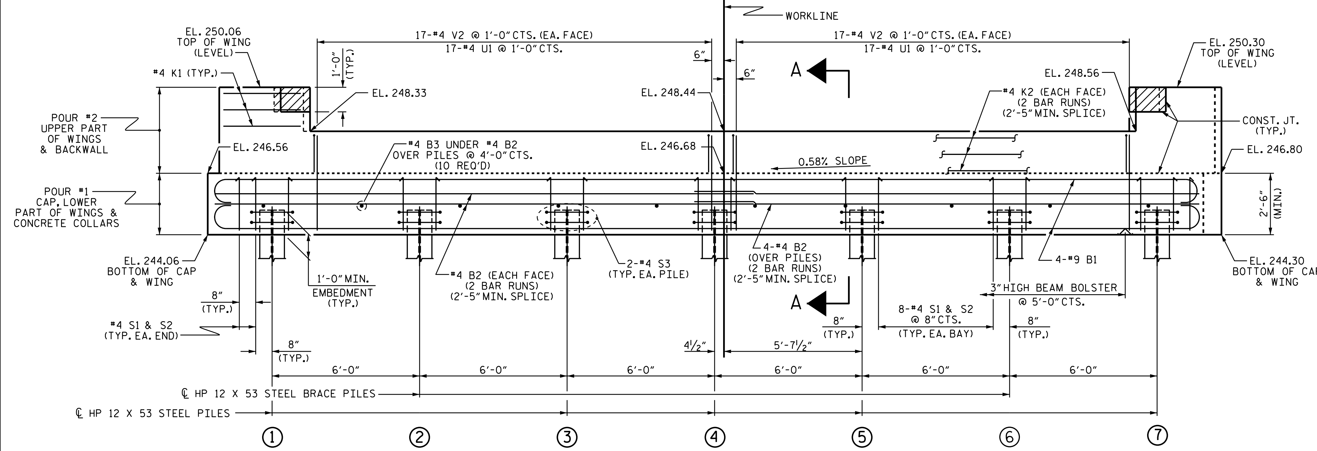
ELEVATION
