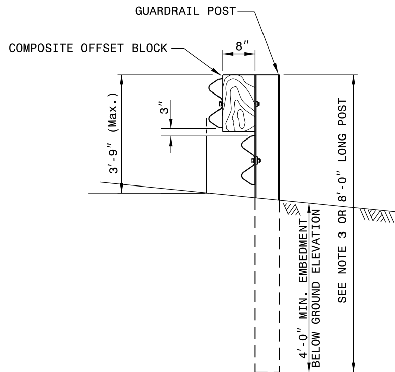
ELEVATION
