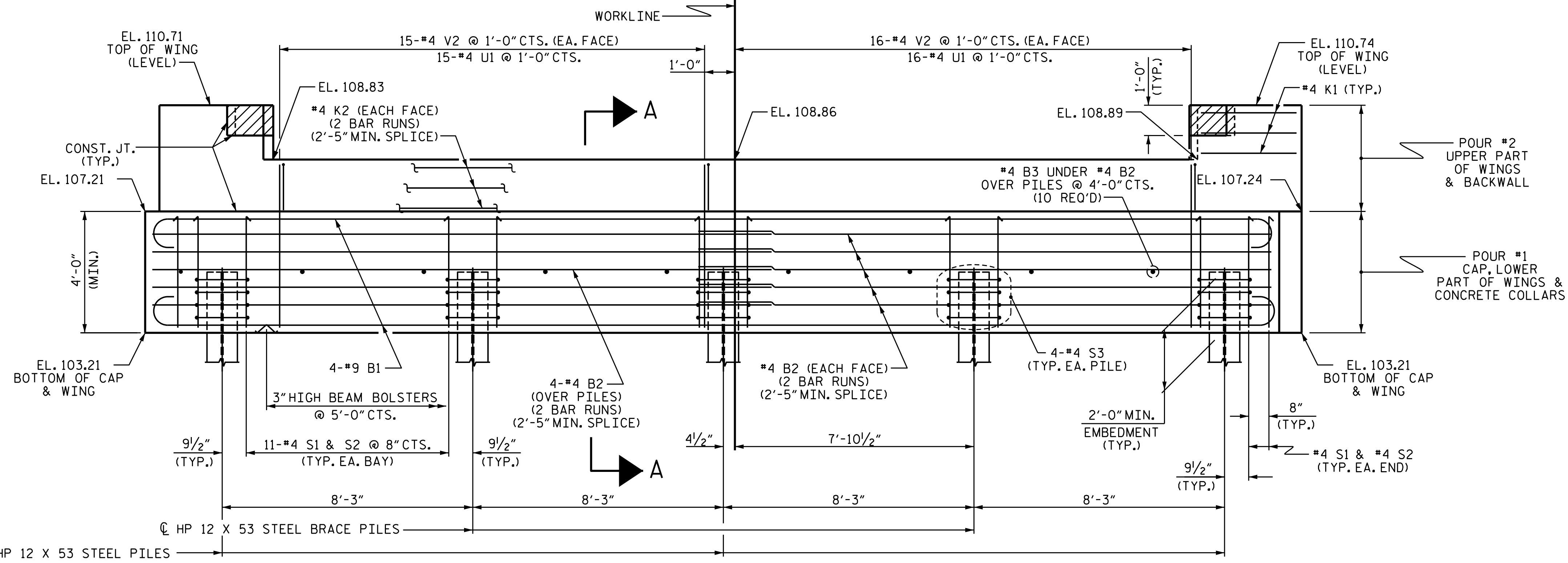
ELEVATION
