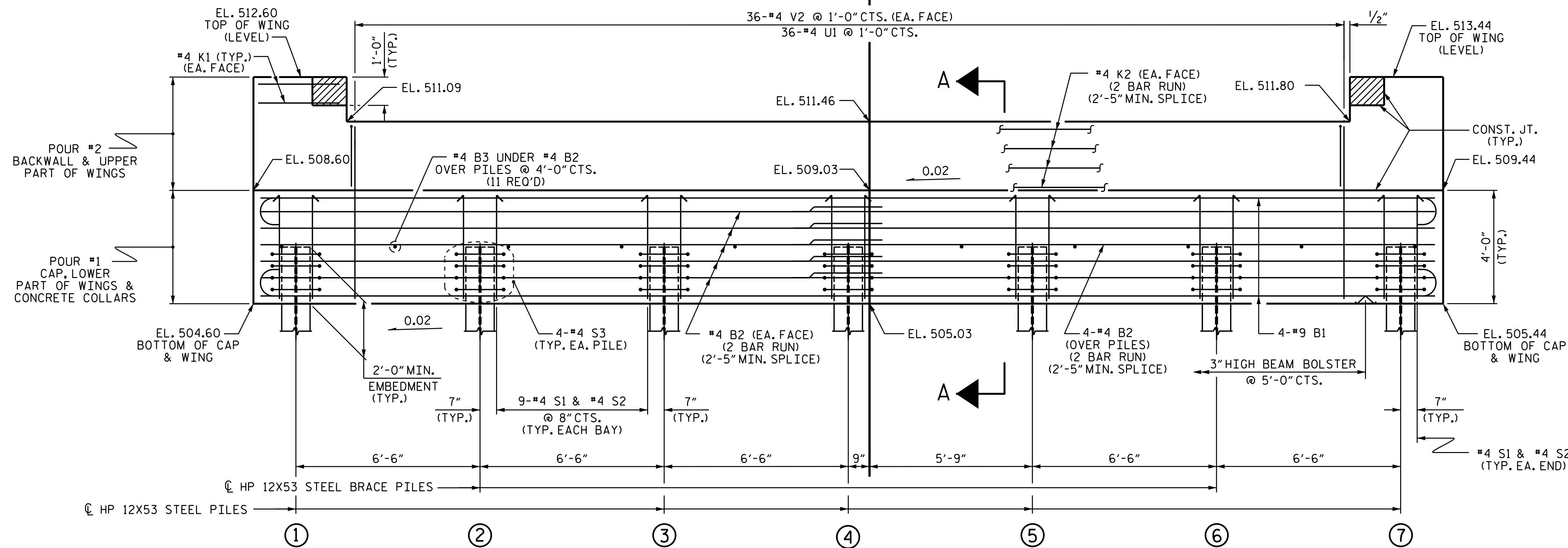
ELEVATION
