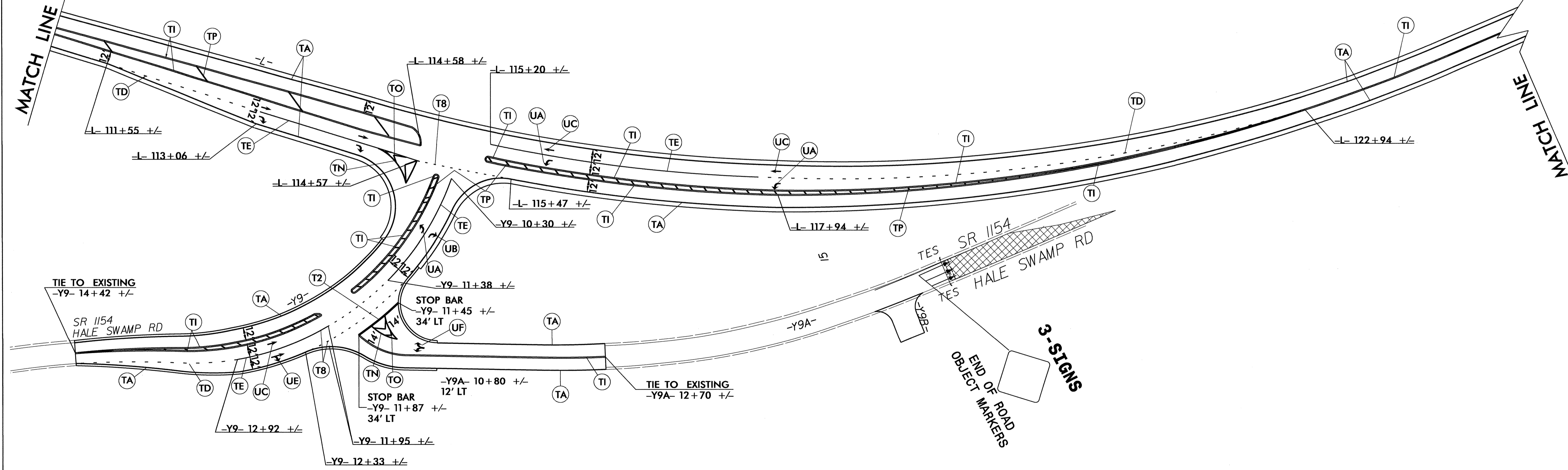
PAVEMENT MARKING DETAIL -L- STA. 111+00 TO STA. 125+00
