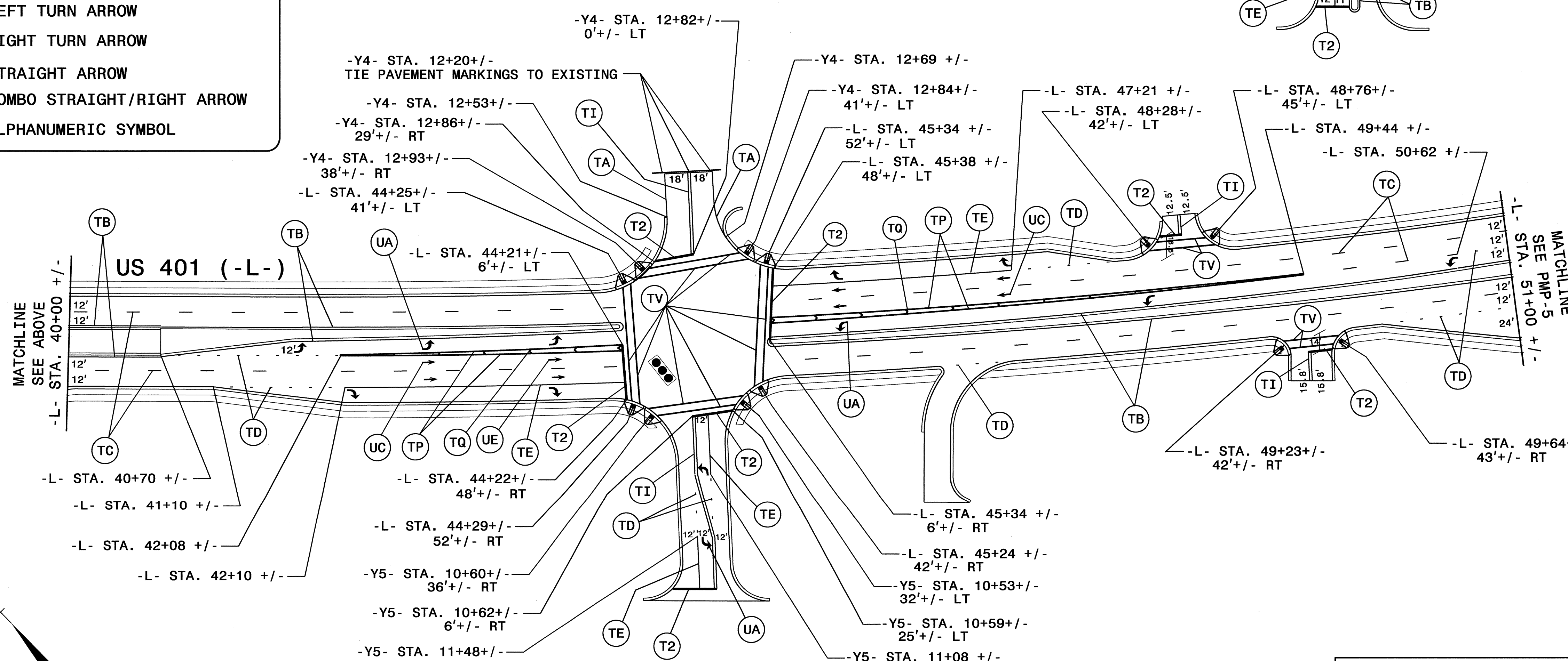
PAVEMENT MARKING DETAILS -L- STA. 29+00.00 TO STA. 51+00.00
