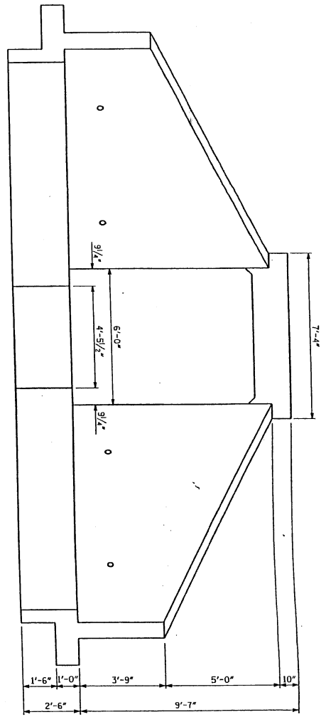
END ELEVATION
