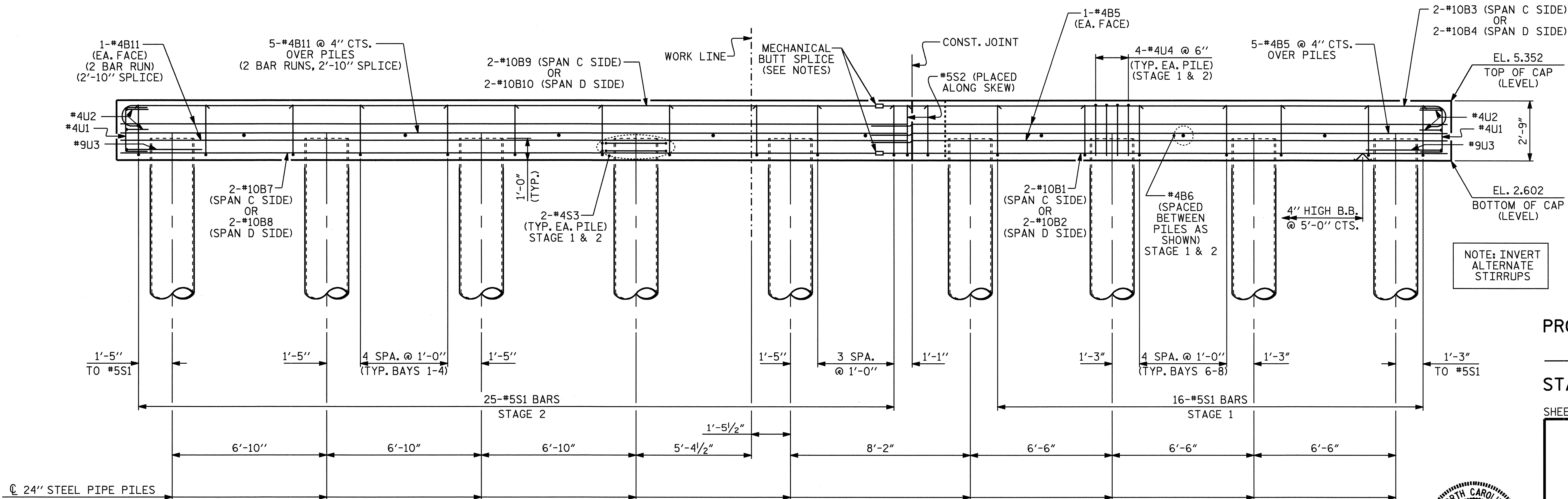
ELEVATION
