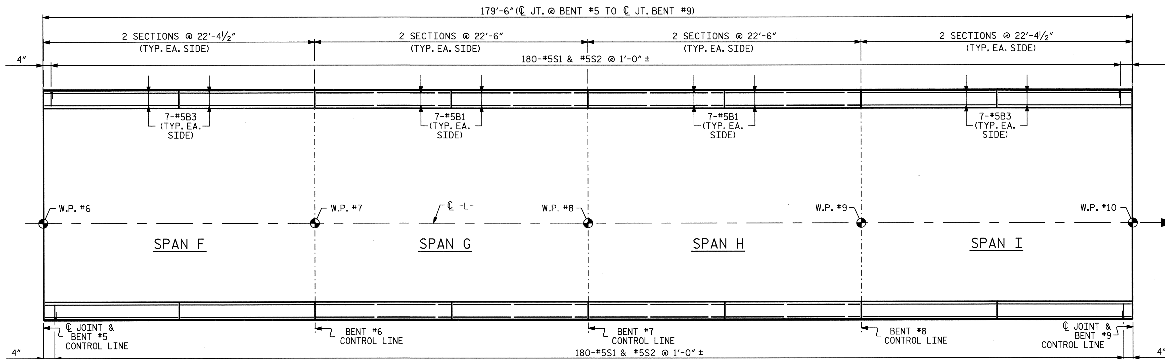
PLAN - SPANS F-I
