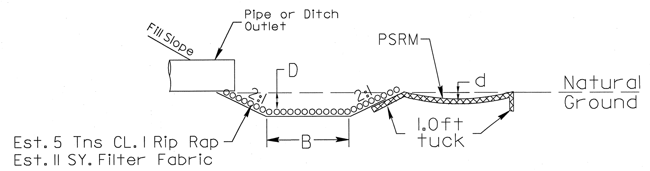
SECTION A-A
