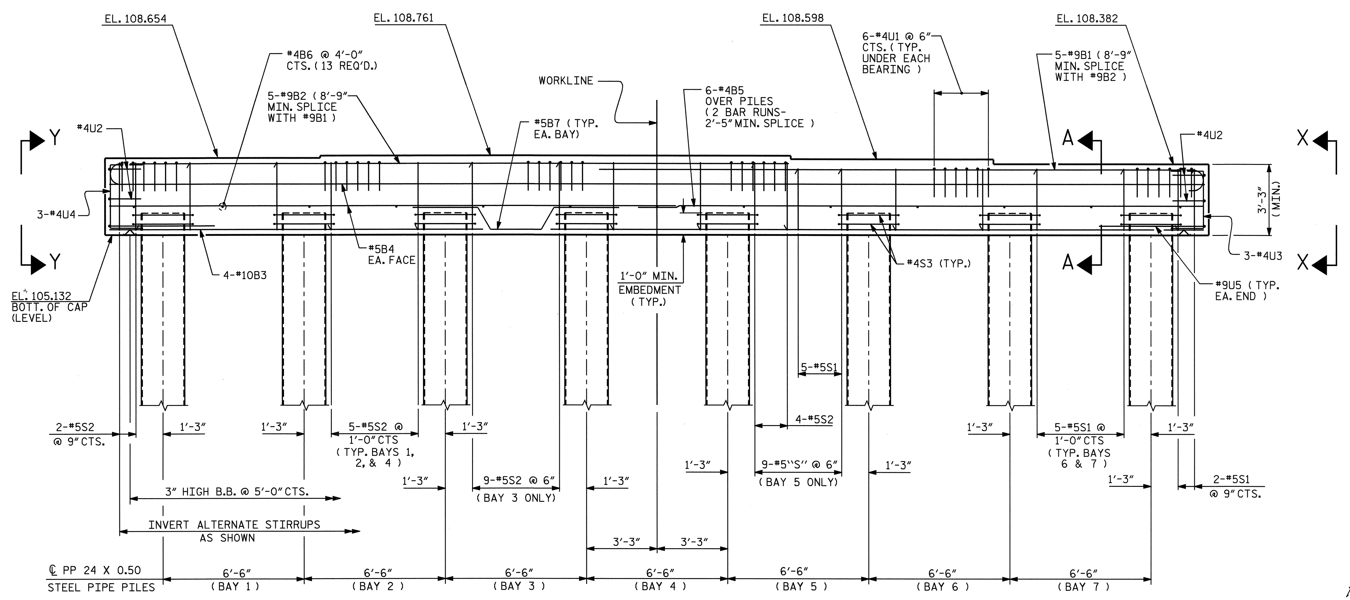
ELEVATION
