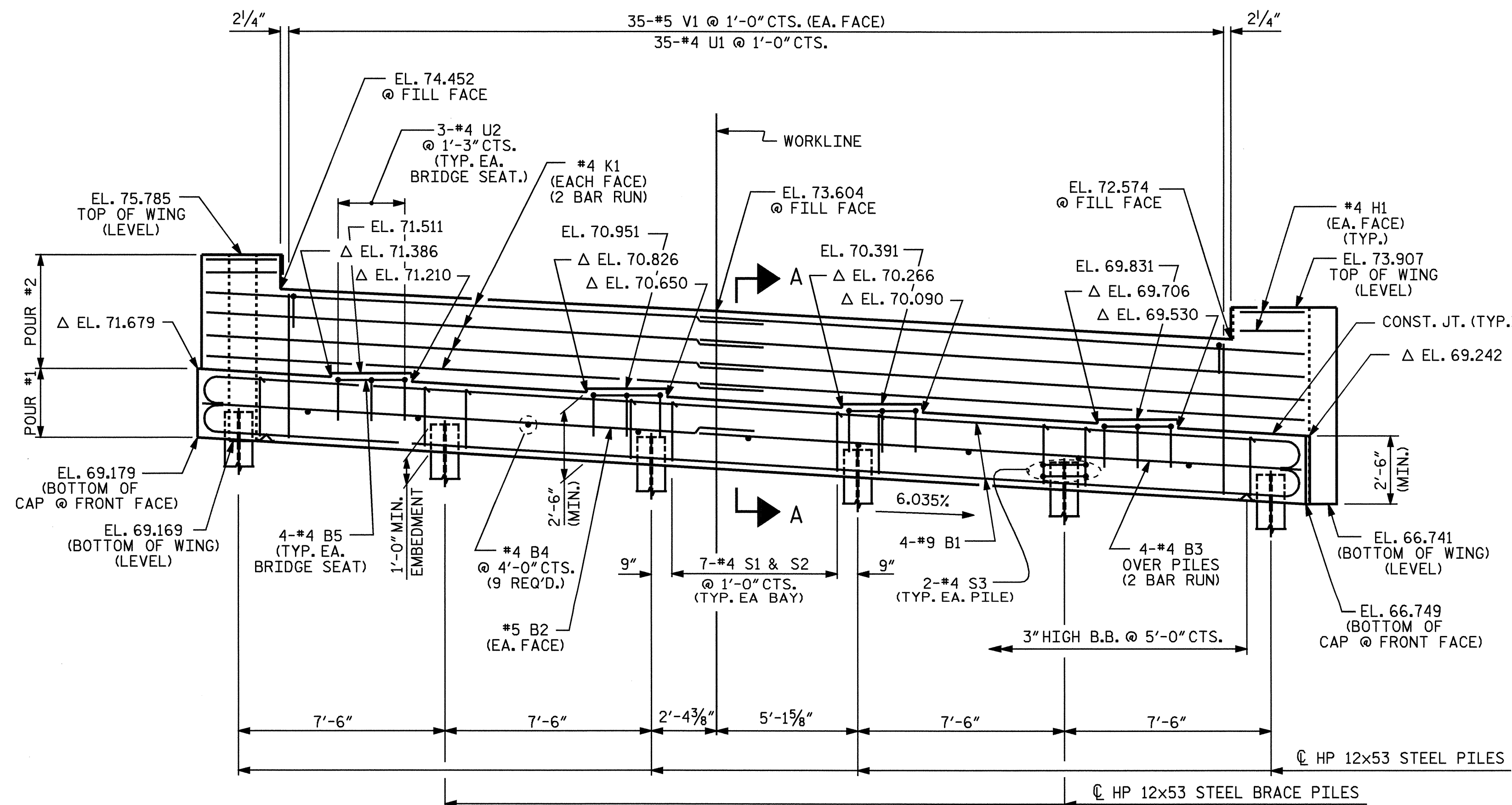
ELEVATION
