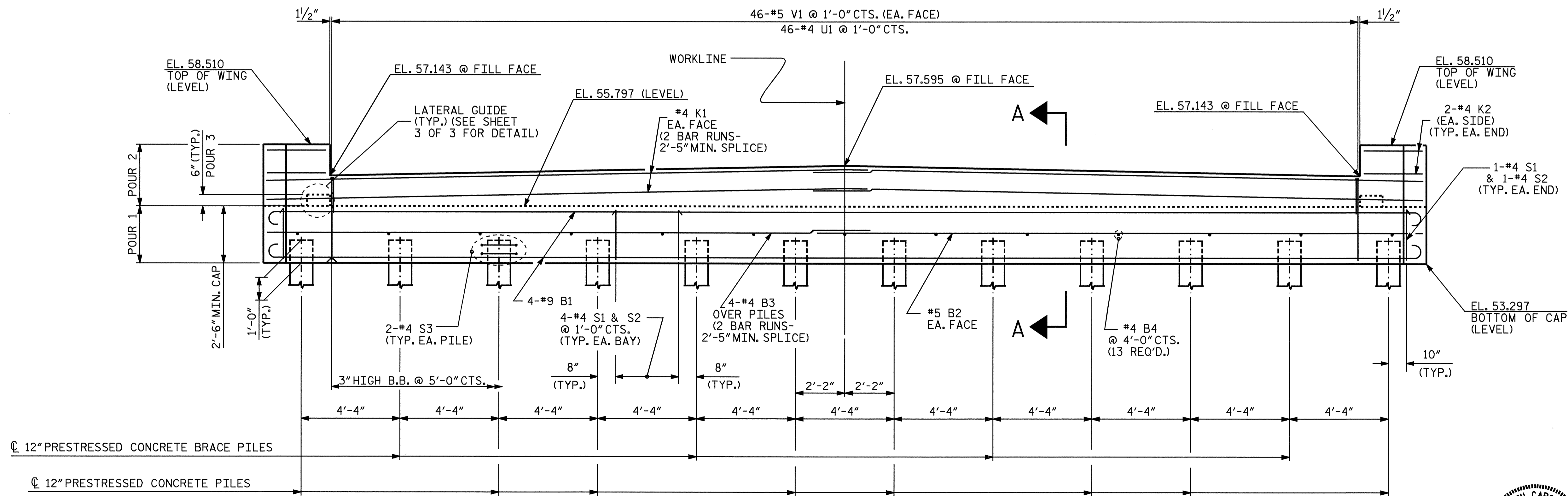
ELEVATION
