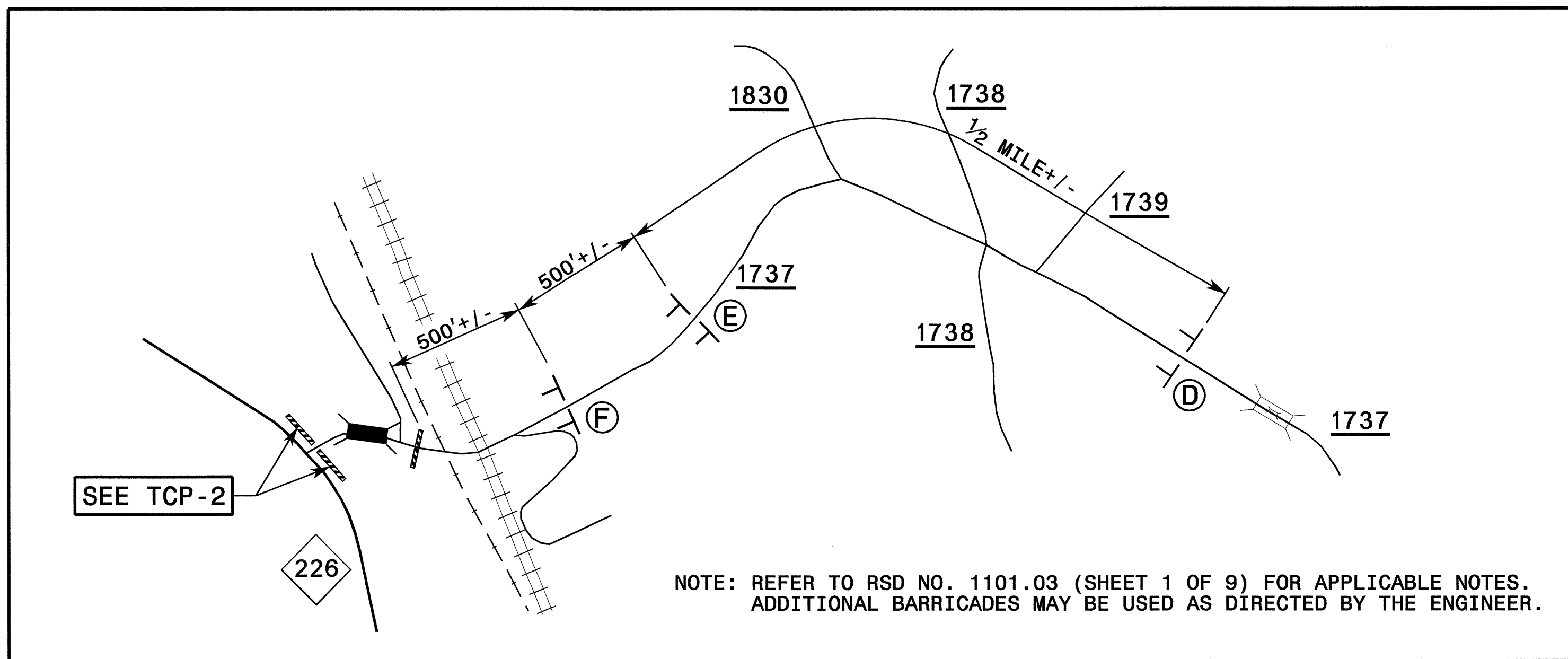
INSET "A"
