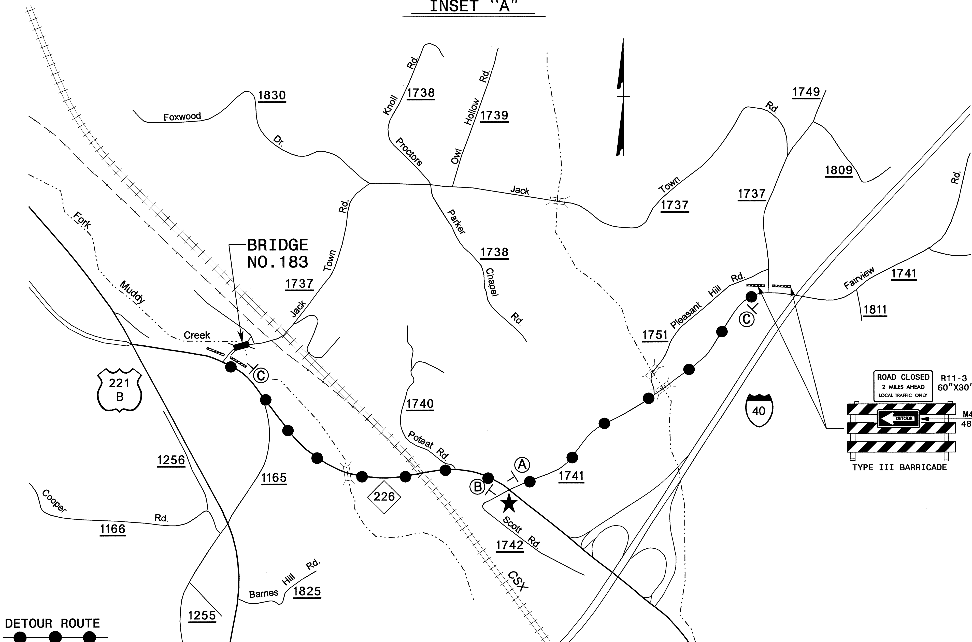
INSET "A"
