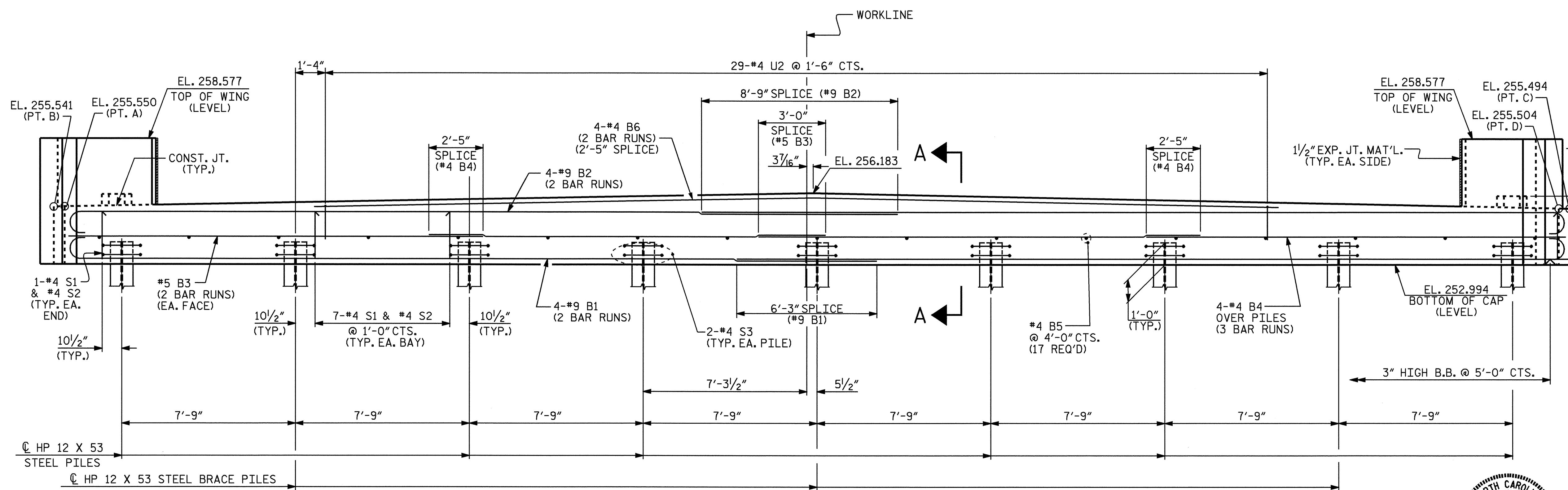
ELEVATION
