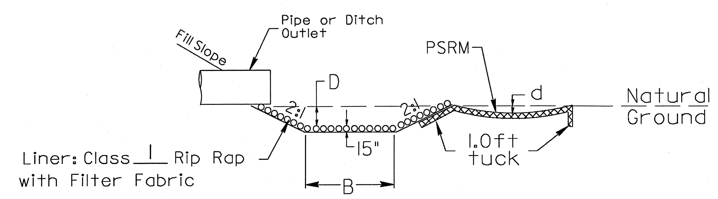
SECTION A-A
