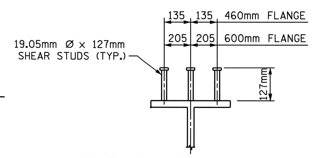
SHEAR STUD DETAILS
