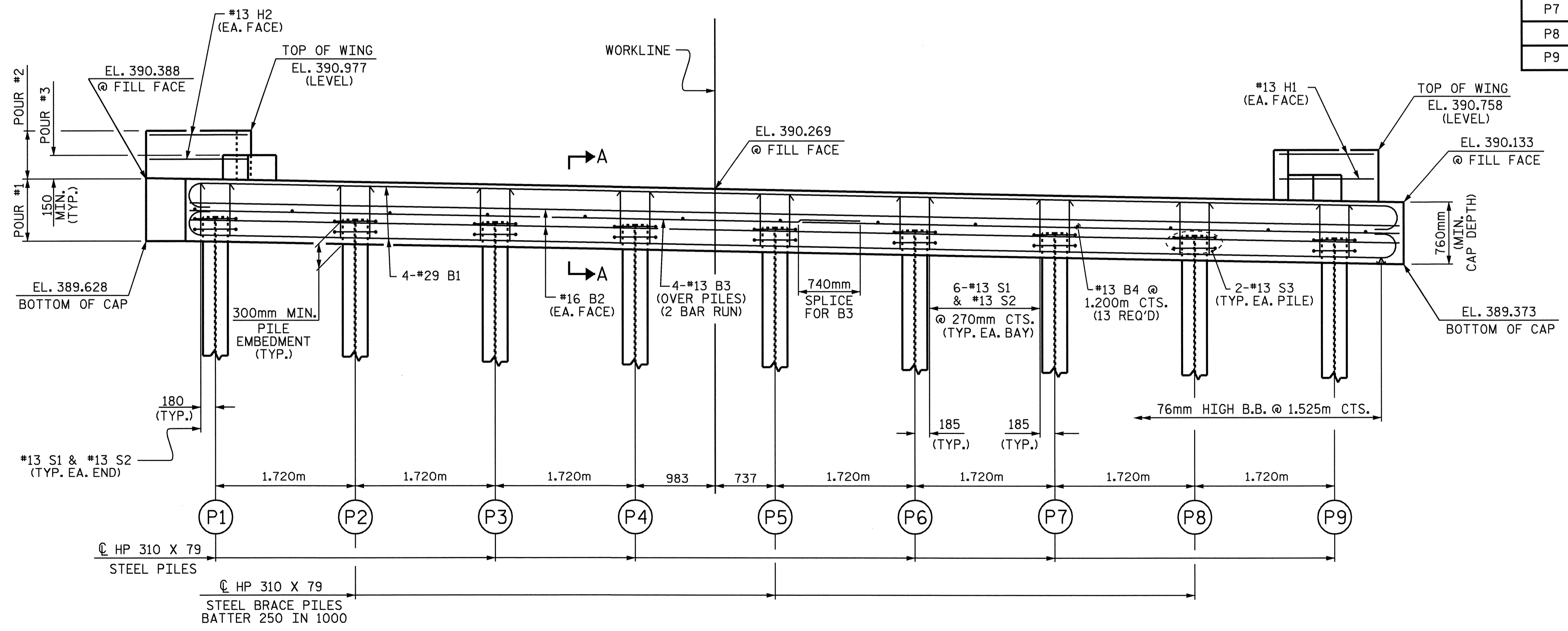
ELEVATION
