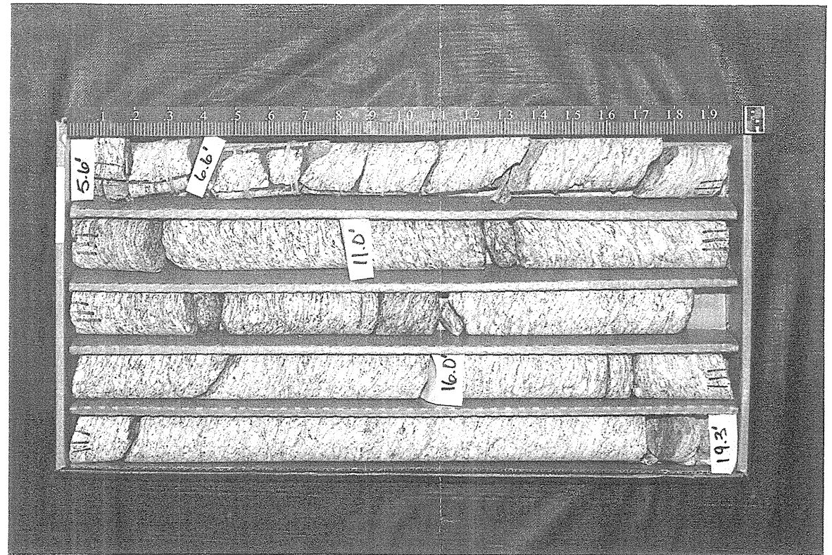
BORING EB1-A STA. 14+37 -L- @ 15.0 LEFT BOX 1 of 2
