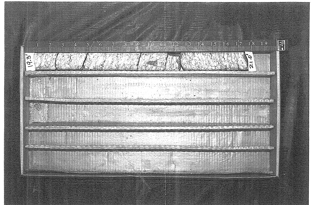
BORING EB1-A STA. 14+37 -L- @ 15.0 LEFT BOX 2 of 2
