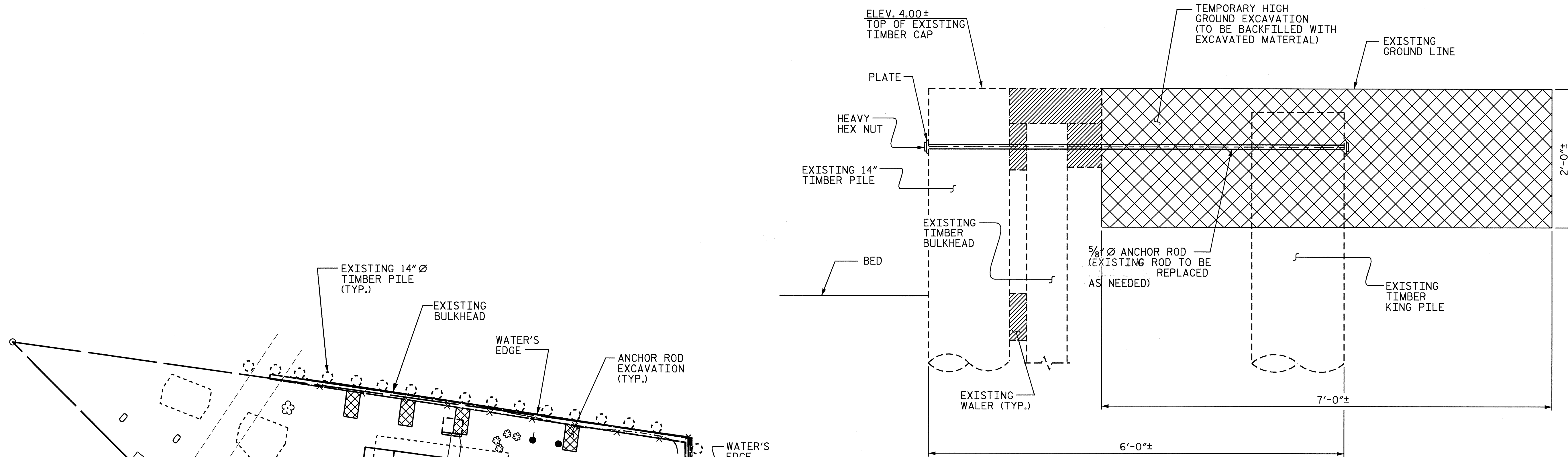
SECTION A-A
