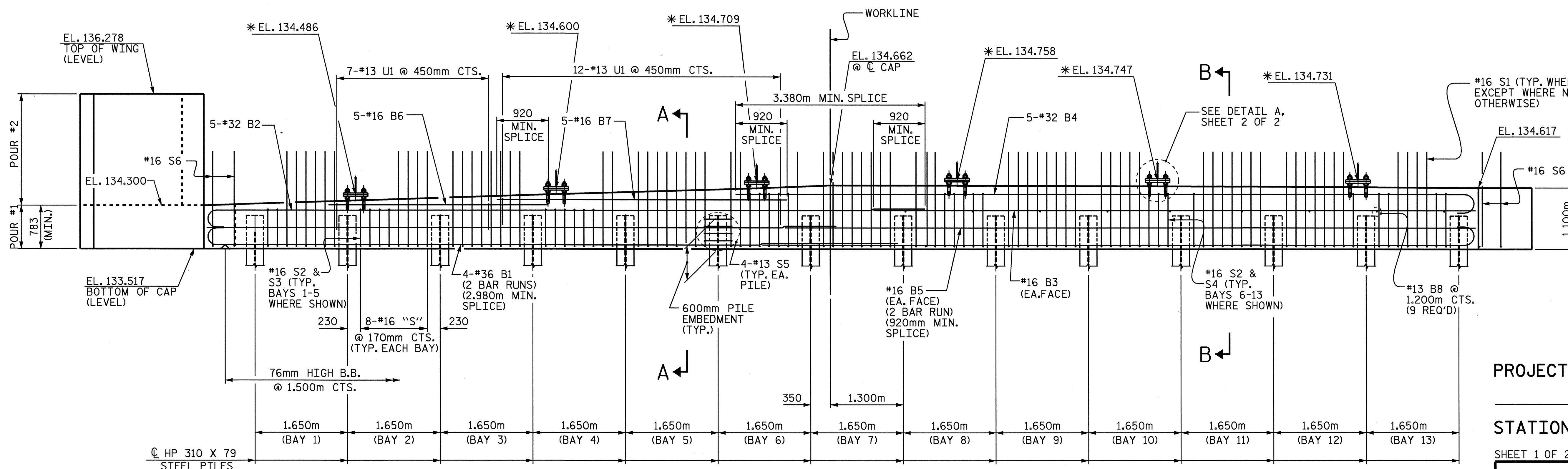
ELEVATION
