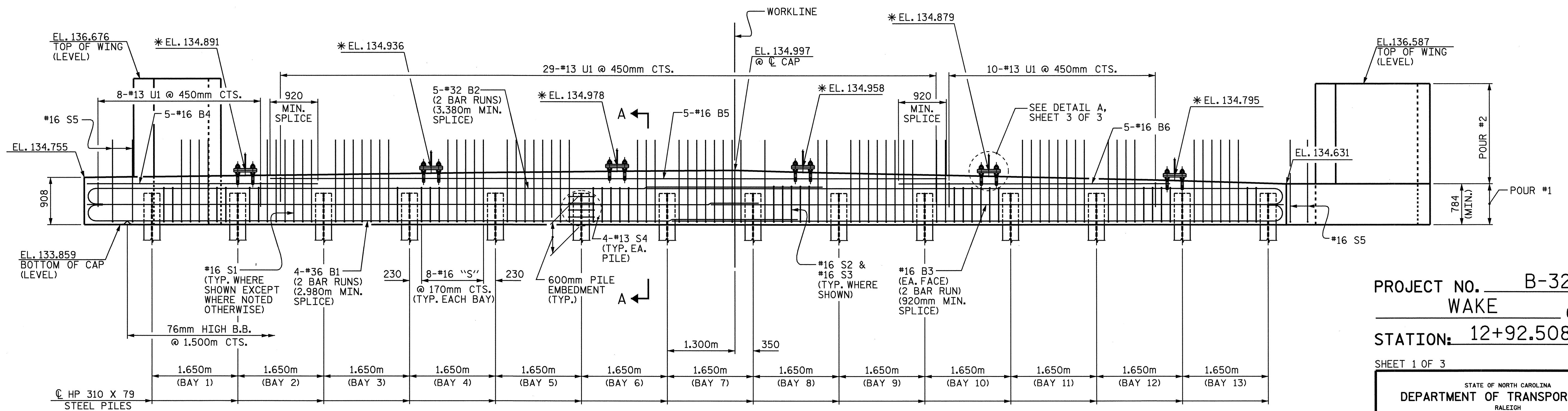
ELEVATION
