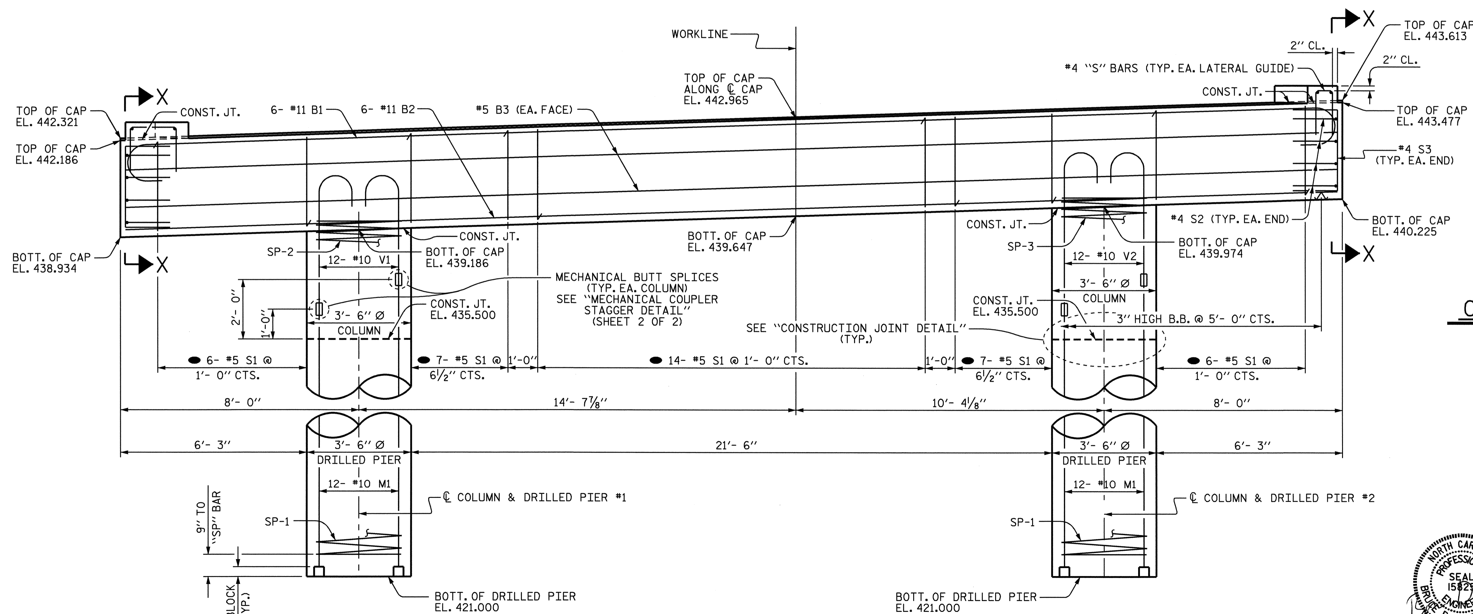
ELEVATION
