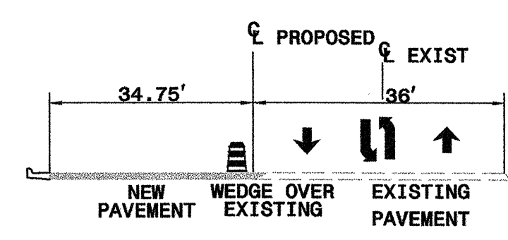
SECTION A-A -L- STA 16+00
