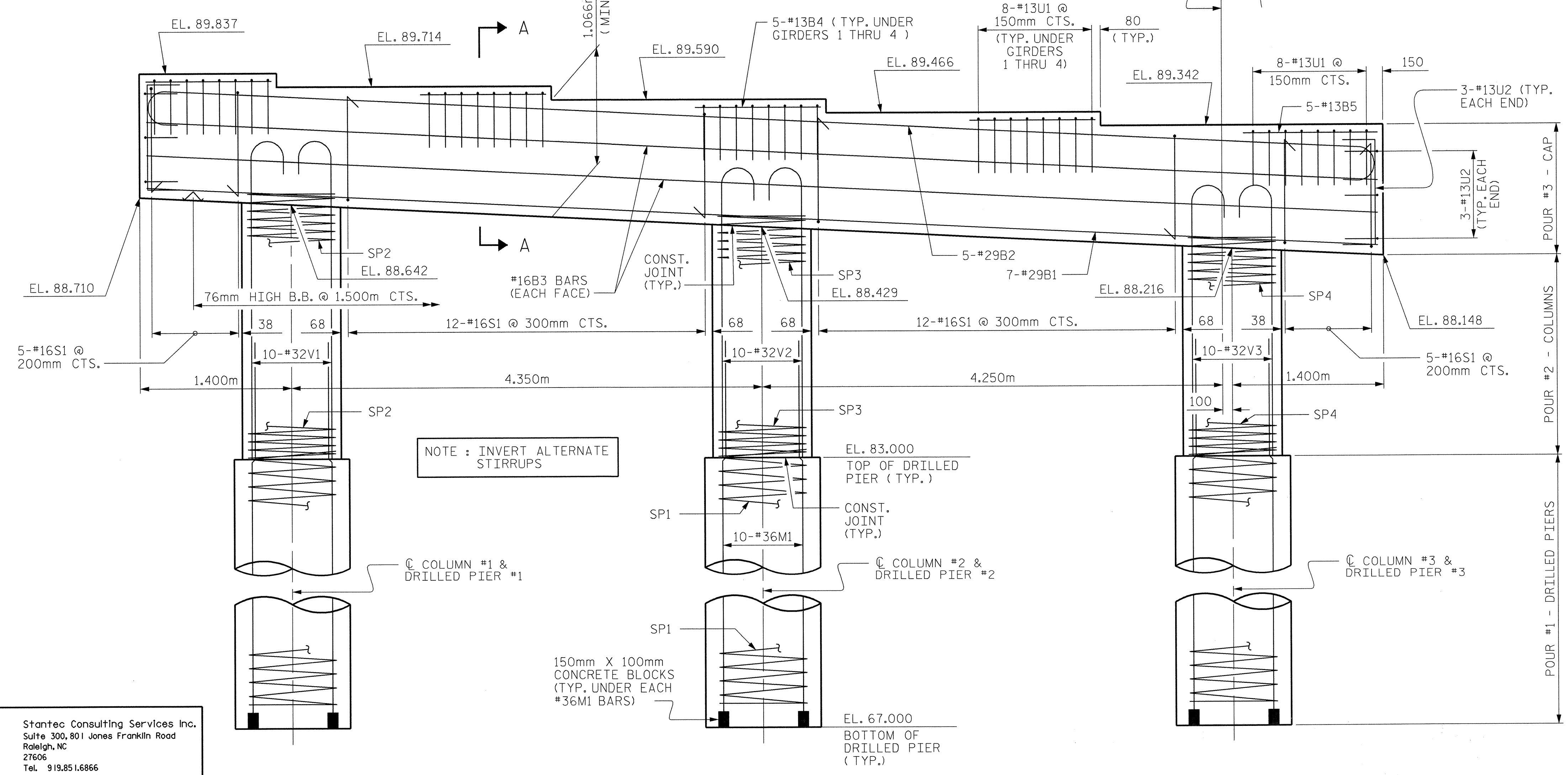
ELEVATION
